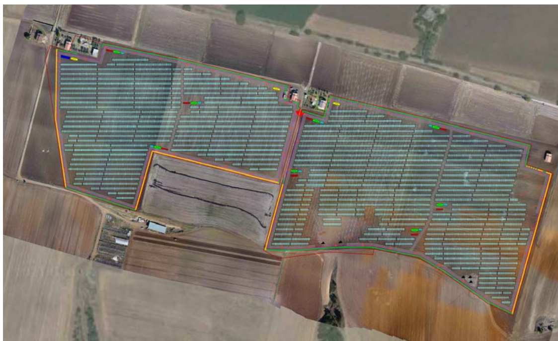
Figura 121: Layout dell'impianto fotovoltaico
