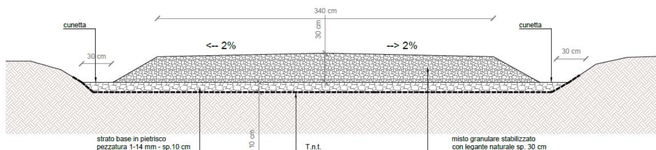
Figura 38: Viabilità tipo
