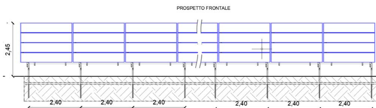
Figura 28 Struttura di sostegno – Prospetto Frontale
