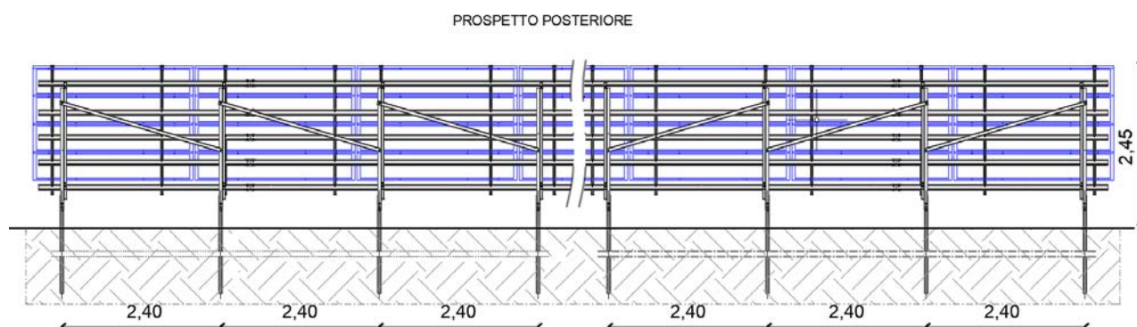
Figura 27: Struttura di sostegno – Prospetto Posteriore
