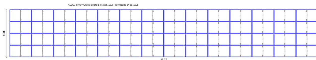
Figura 29 - Struttura di sostegno 4x14 moduli- 2 Stringhe - Pianta
