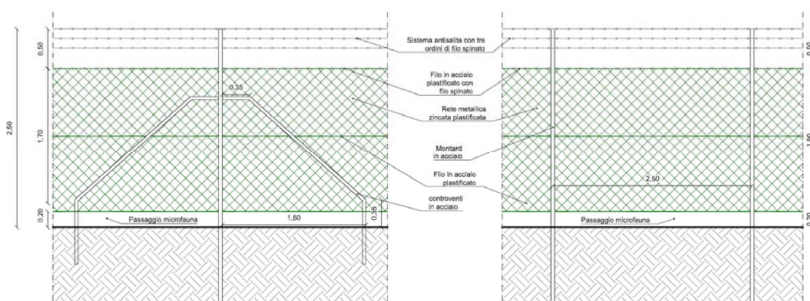
Figura 39: Recinzione tipo
