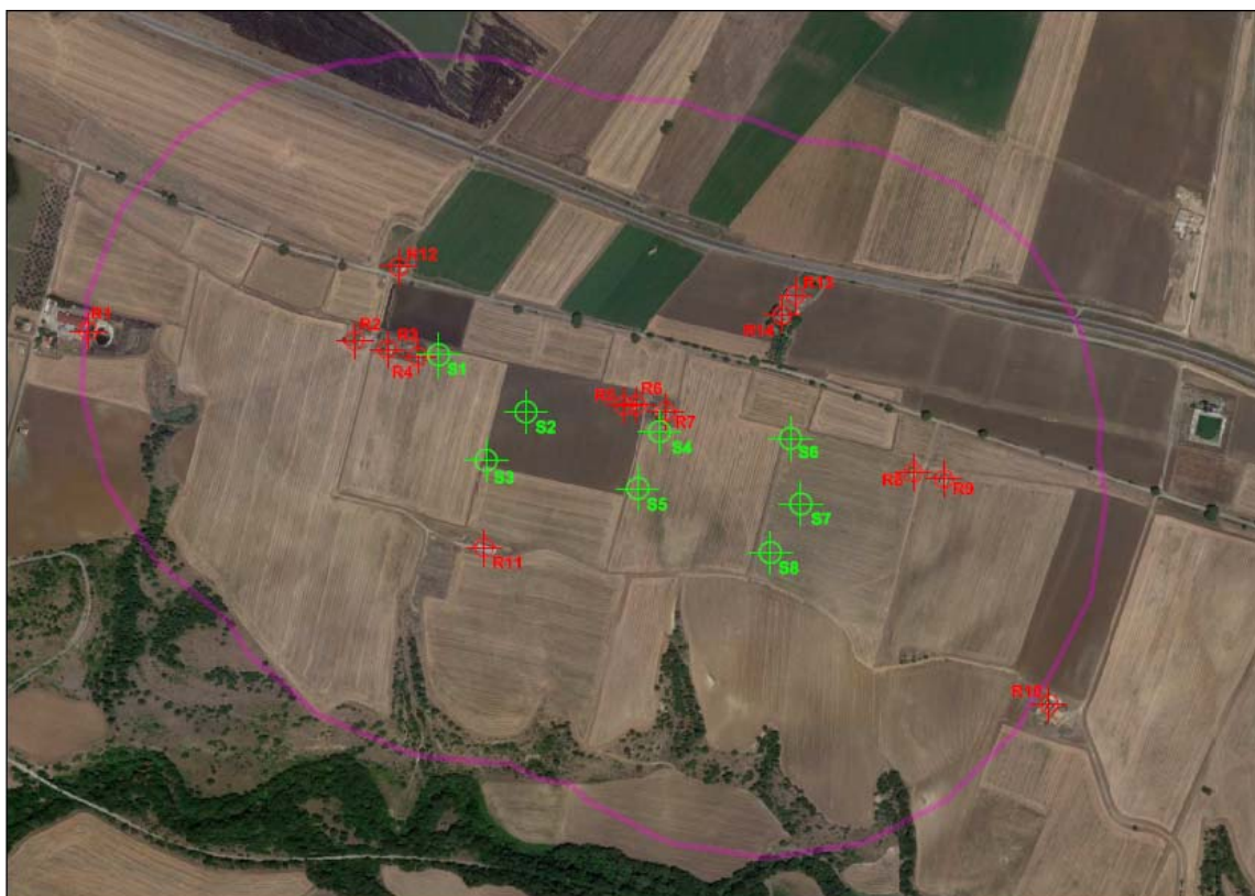
Figura 104: Planimetria con ubicazione dei Ricettori (R i ) e delle Sorgenti (S i )
