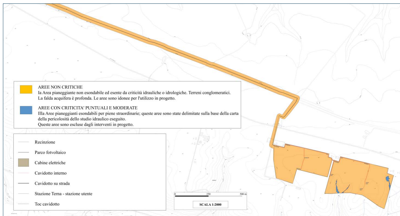
Figura 99: Stralco della Carta della pericolosità e criticità geologica e geomorfologica
