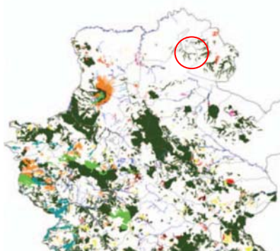
Figura 100: Stralcio Carta Forestale Regionale
