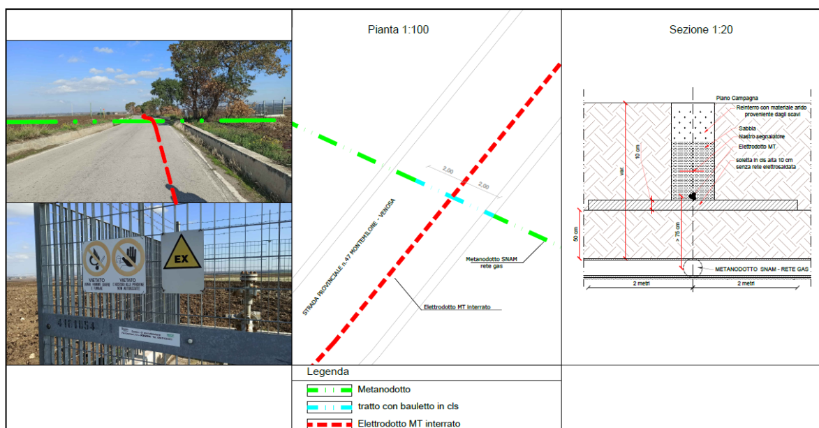
Figura 19: Foto opere e progettazione risoluzione Interferenza I.04
