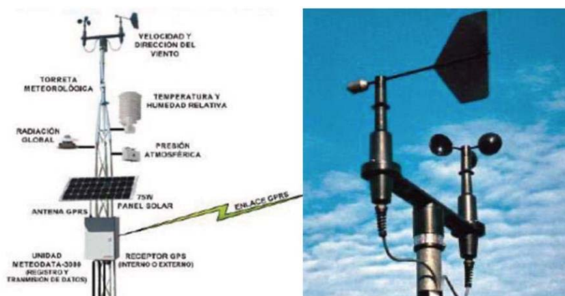
Figura 37: Stazione meteorologica
