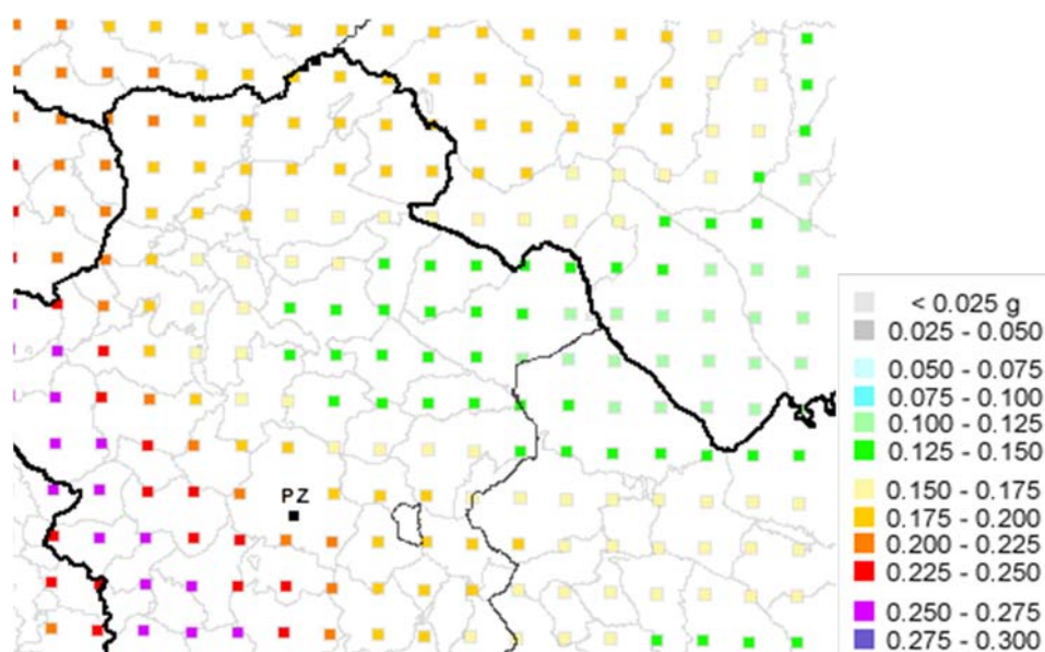
Figura 97: Stralcio della Mappa di pericolosità sismica ( T_r = 475 anni) - Fonte INGV.
