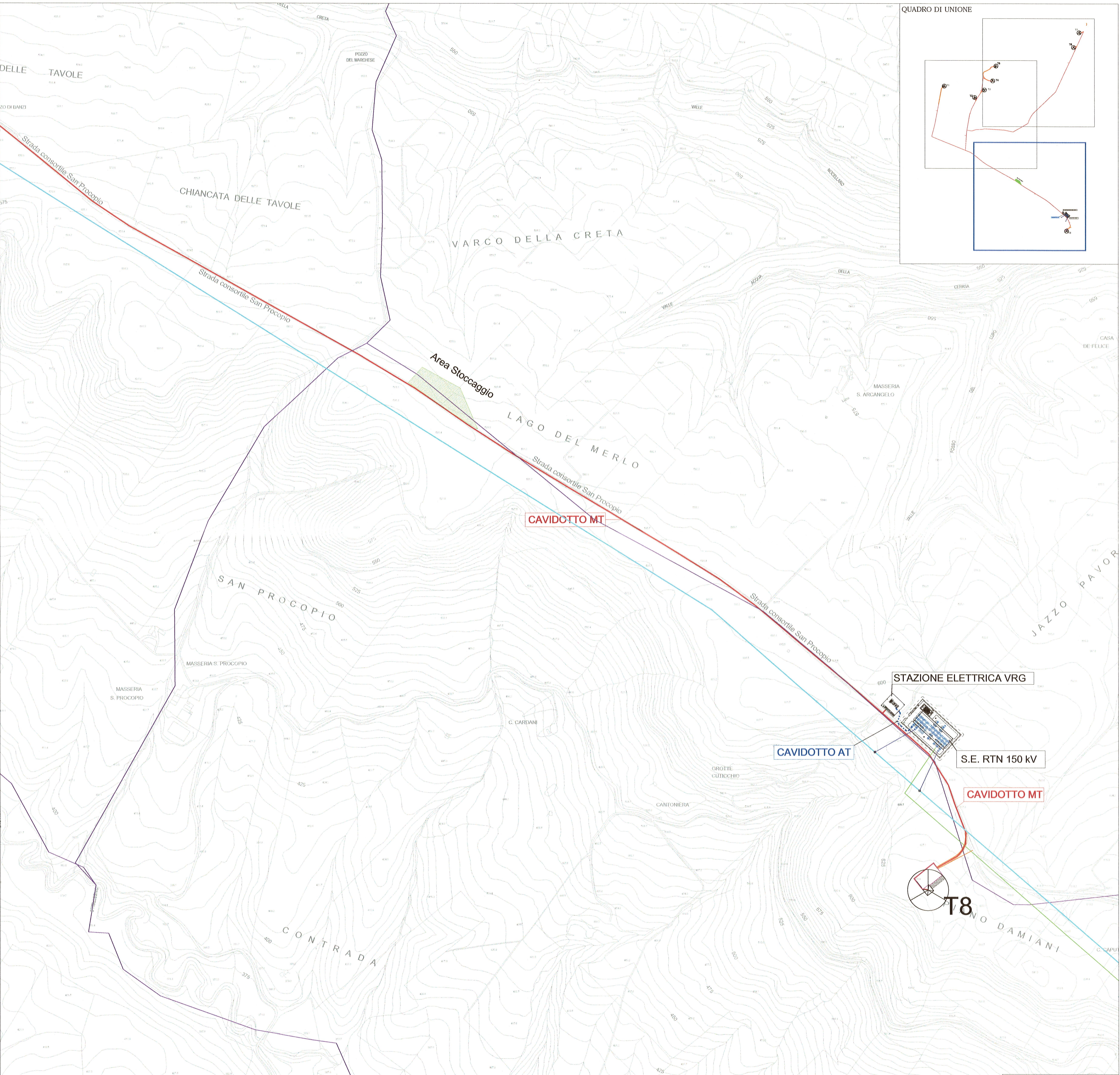
PLANIMETRIA CTR - scala 1:5000
