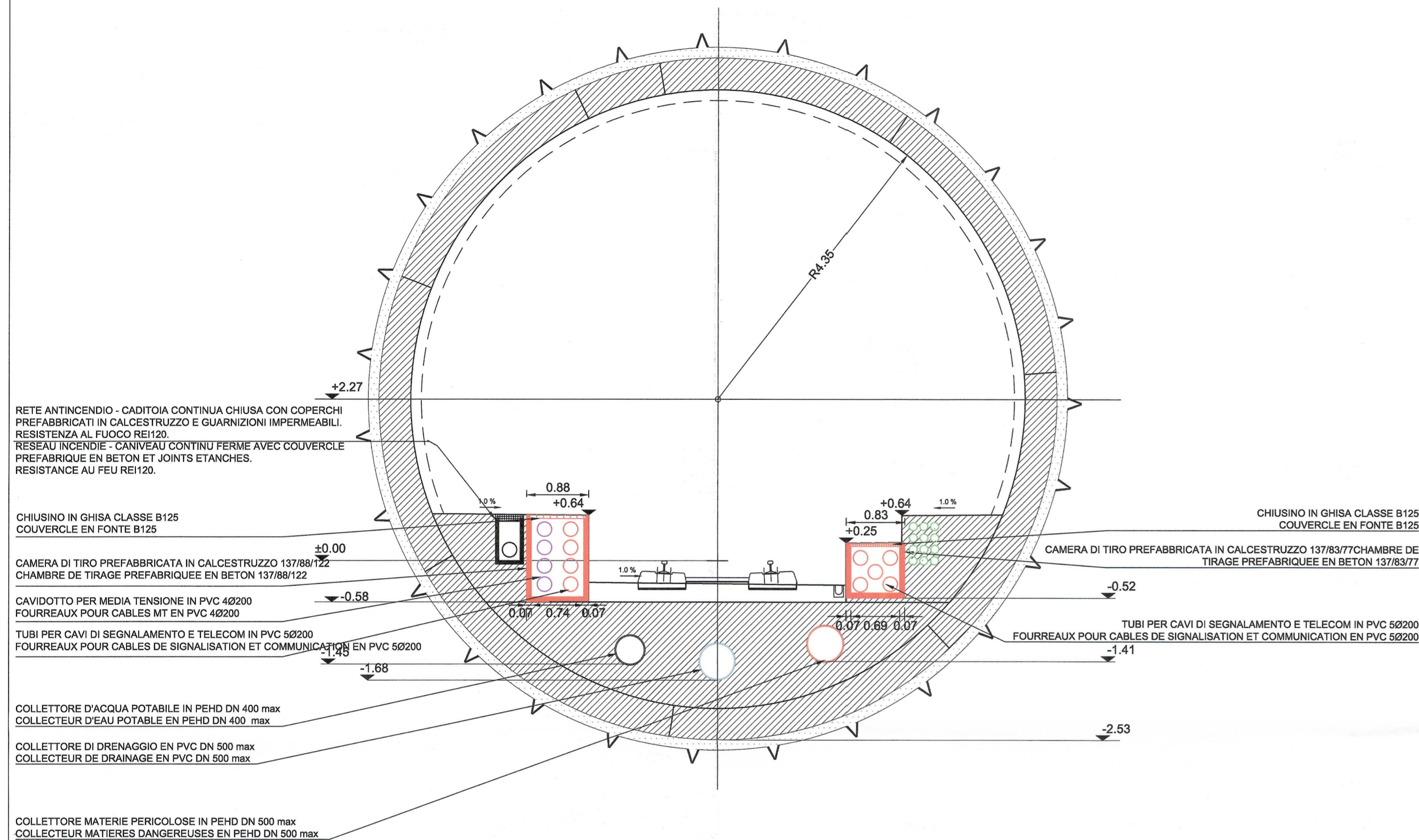
SEZIONE A-A / COUPE A-A
