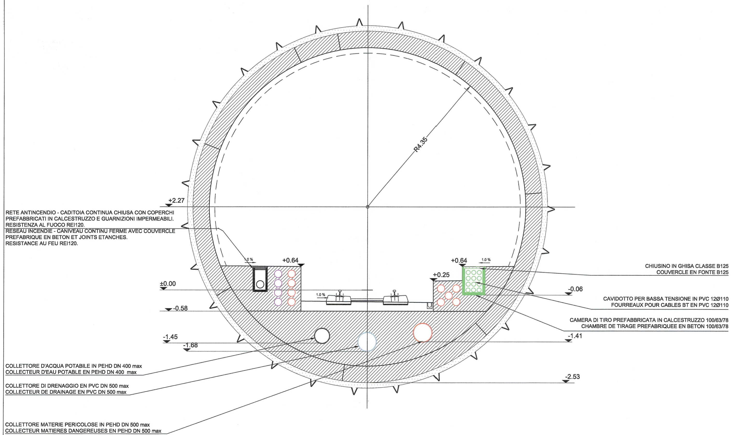
SEZIONE B-B / COUPE B-B
