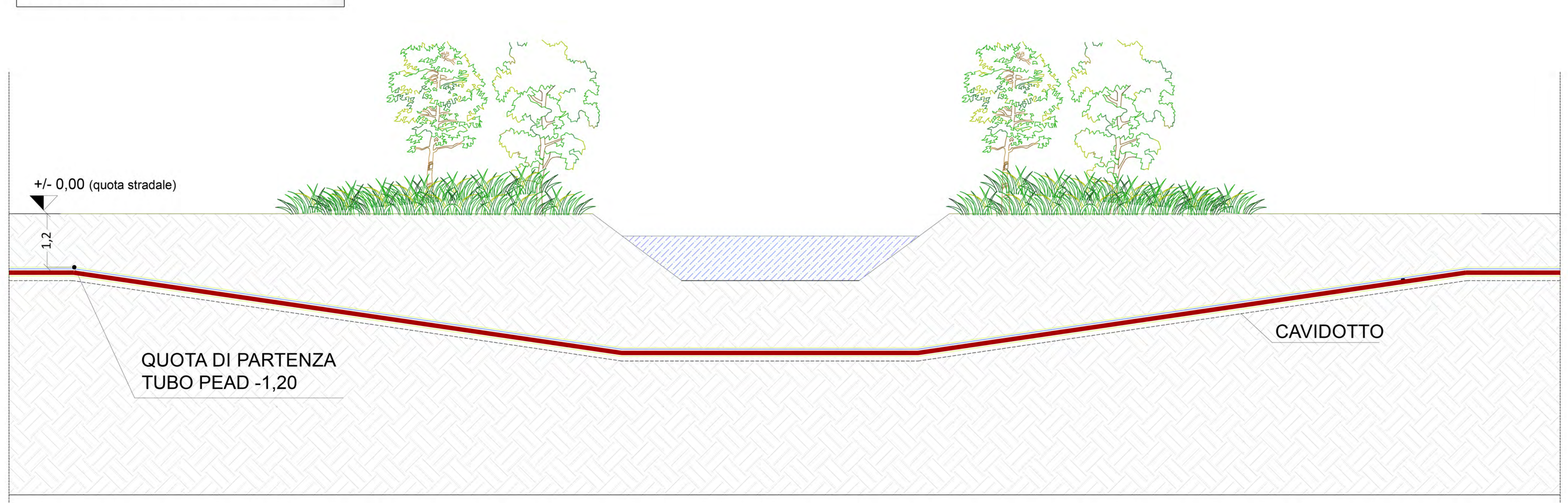
Sezione tipo delle interferenze scala 1:50
