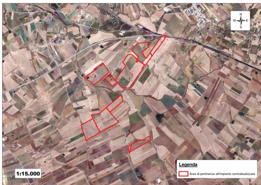
Figura 1 – Area di progetto dell'impianto fotovoltaico su ortofoto.
