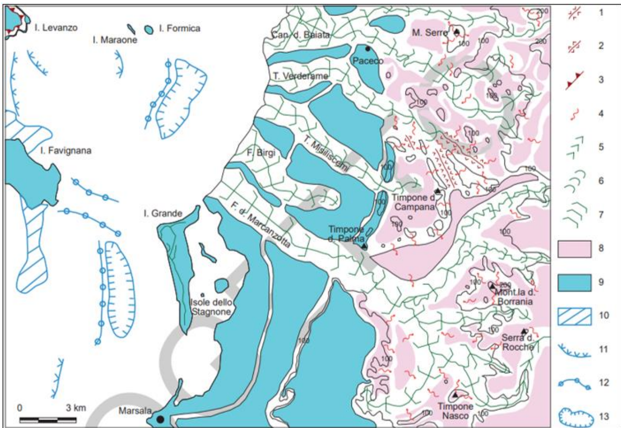
Schema geomorfologico dell'area del Foglio "Paceco"
