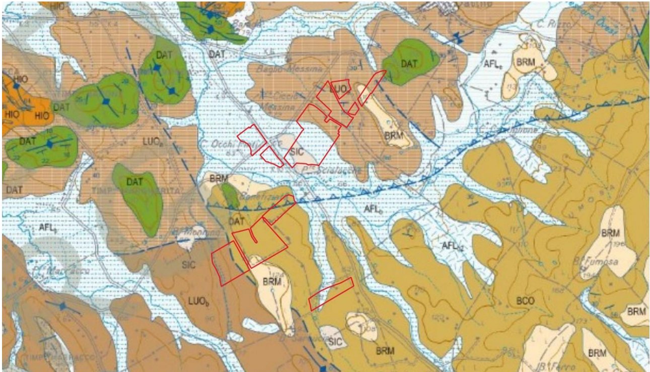
CARTA GEOLOGICA
