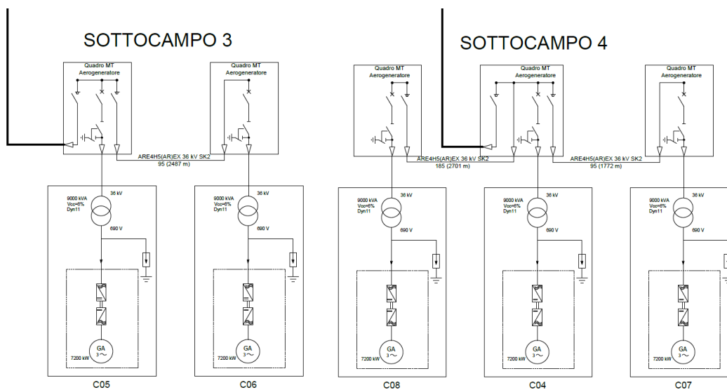
Schema a blocchi del parco eolico GRUPPO 3 e GRUPPO 4
