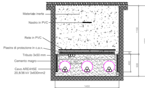
TIPICO CAVIDOTTO A.T. INTERRATI POSA INTERRATA A TRIFOGLIO SU SEDE STRADALE
