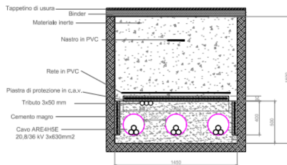
TIPICO CAVIDOTTO A.T. INTERRATI POSA INTERRATA A TRIFOGLIO SU SEDE STRADALE
