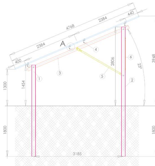
Figura 1- Sezione trasversale del telaio di supporto
