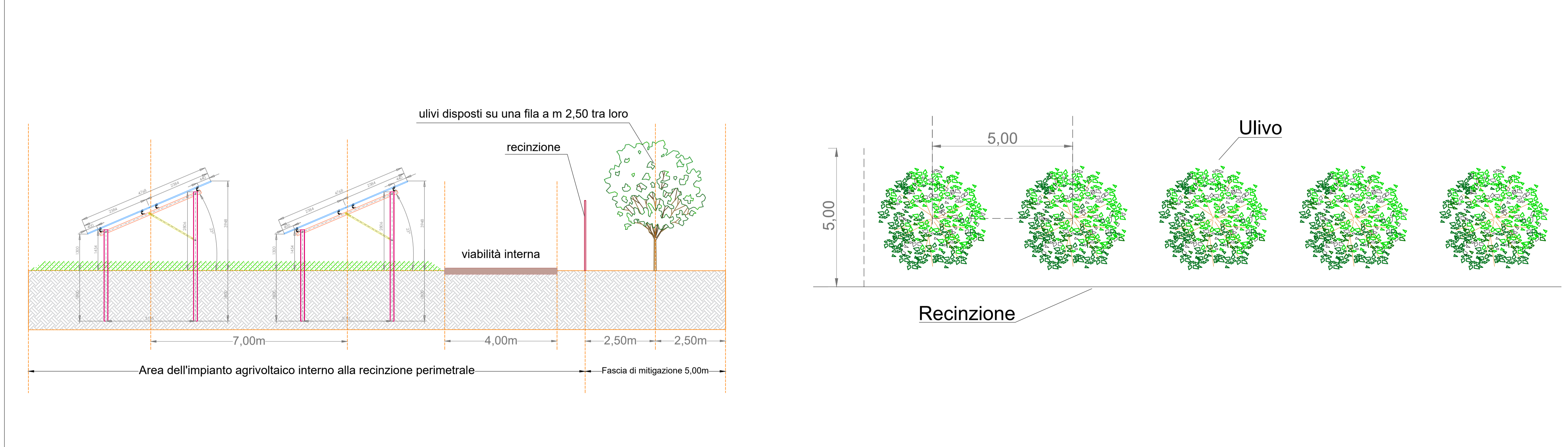
Sezione impianto, colture interfila e opere di mitigazione visiva Confine tra l'impianto agrivoltaico e altre proprietà - Uliveto intensivo Pianta opere di mitigazione visiva Confine tra l'impianto agrivoltaico e altre proprietà - Uliveto intensivo
