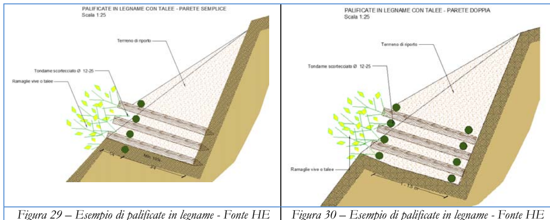
Figura 29 – Esempio di palificate in legname - Fonte HE
