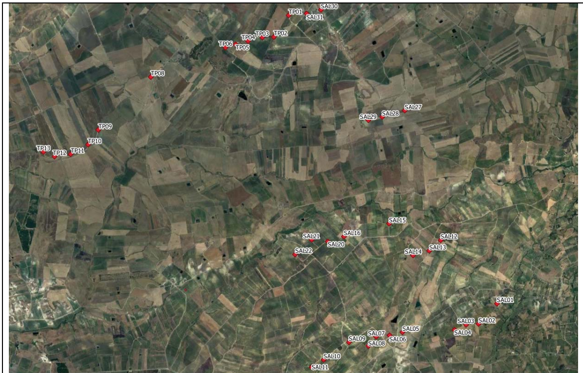
Figura 9 – Layout dell'impianto esistente composto da n. 36 aerogeneratori
