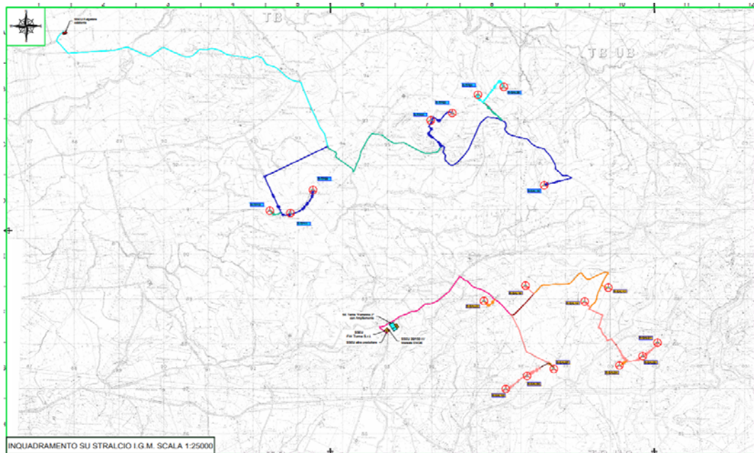
Figura 5- Inquadrimento impianto su IGM 1:25.000
