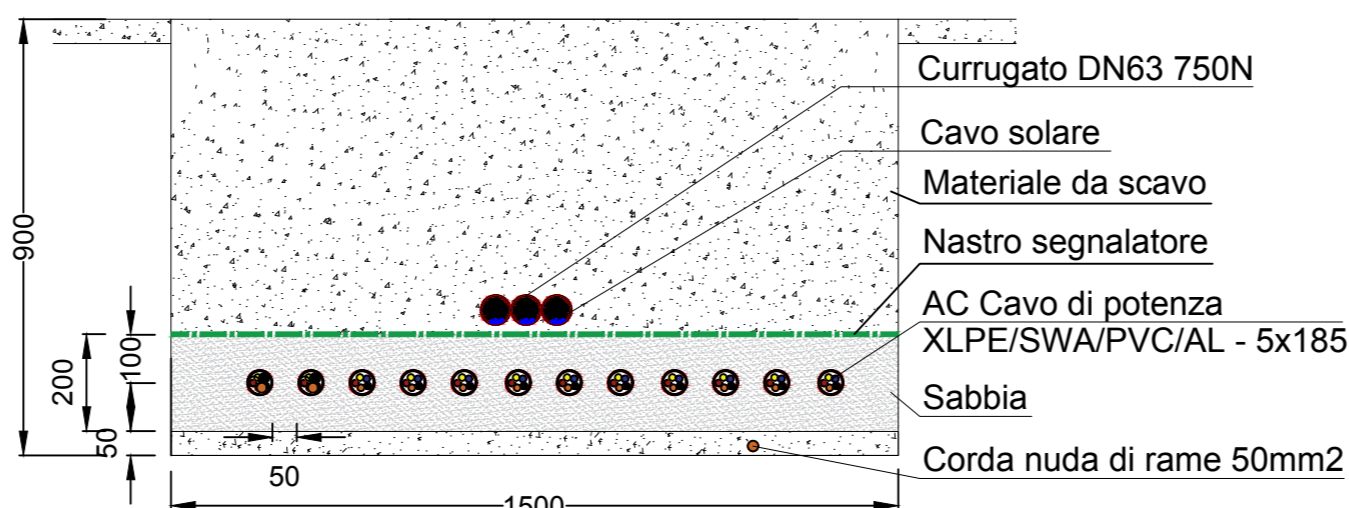
Scavo tipo AC - A3 (fino a 14 circuiti AC e fino a 3 corrugati DN63) Lx1500mm
