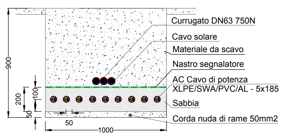
Scavo tipo AC - A2 (fino a 9 circuiti AC e fino a 3 corrugati DN63) Lx900mm
