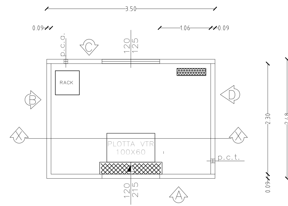
PIANTA
