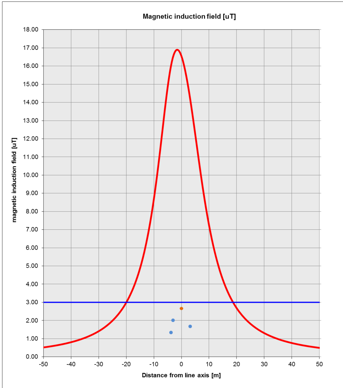
Figura 5.6.2a Andamento dell'Induzione Magnetica in una Sezione Perpendicolare agli Assi della Linea, Calcolata ad 1,5 m dal Suolo nel caso di Franco Minimo (Obiettivo di Qualità pari a 3 microT) – Terna Singola
