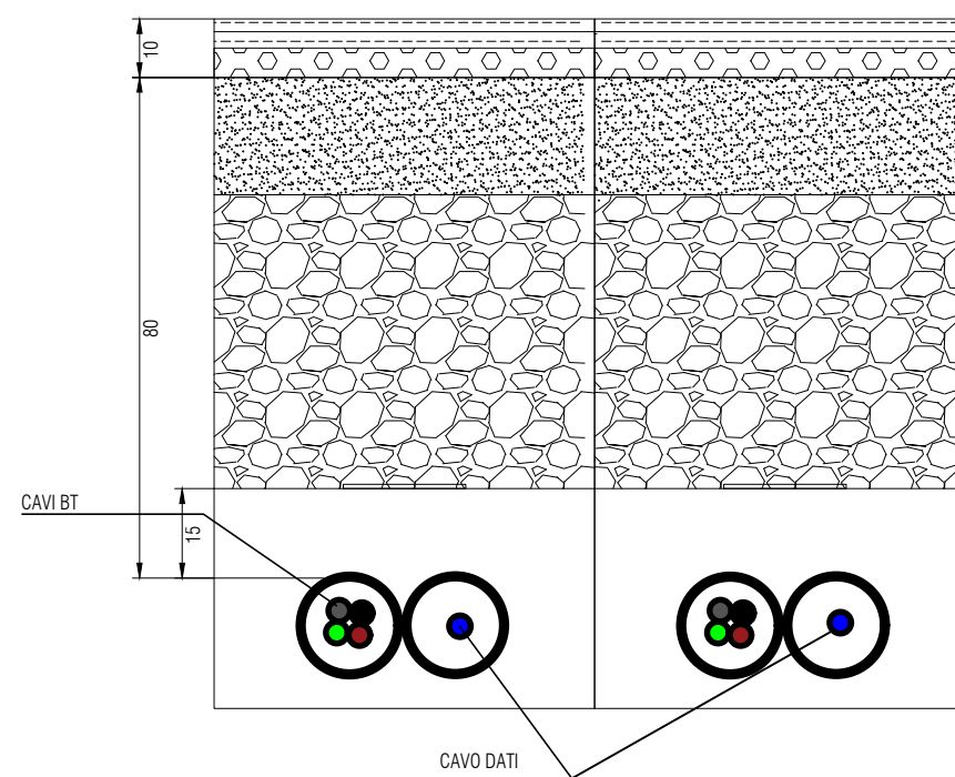
SEZIONE 4-4
