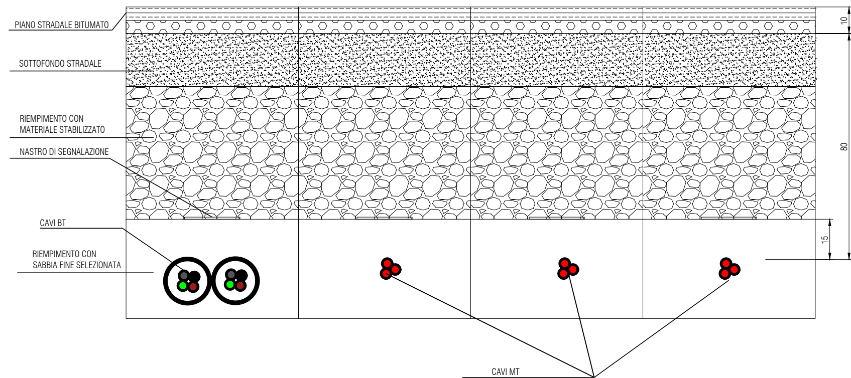
SEZIONE 1-1
