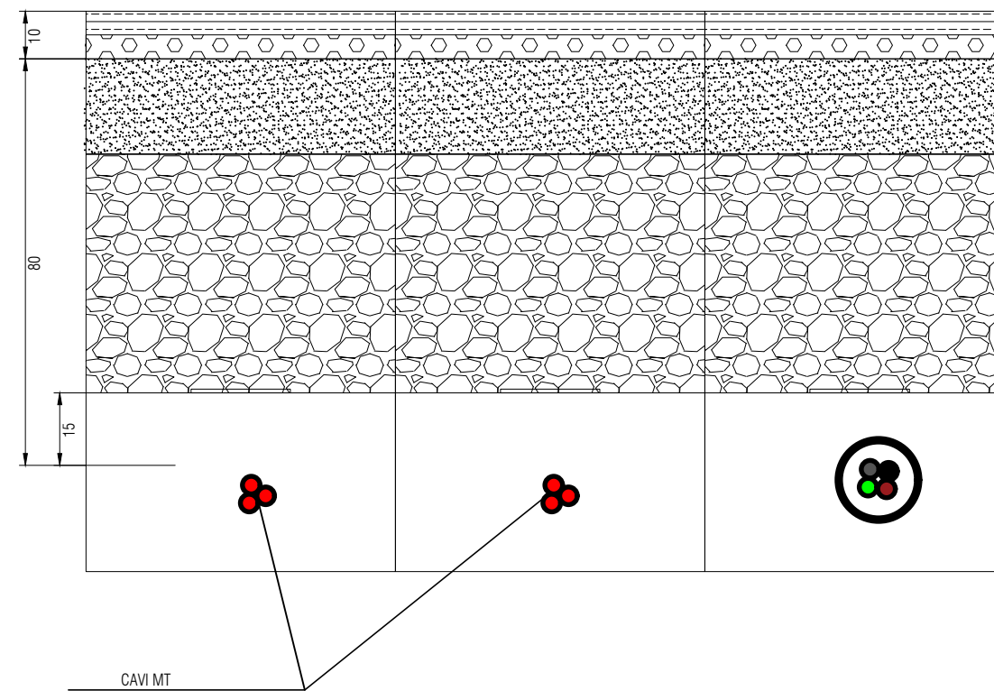
SEZIONE 2-2
