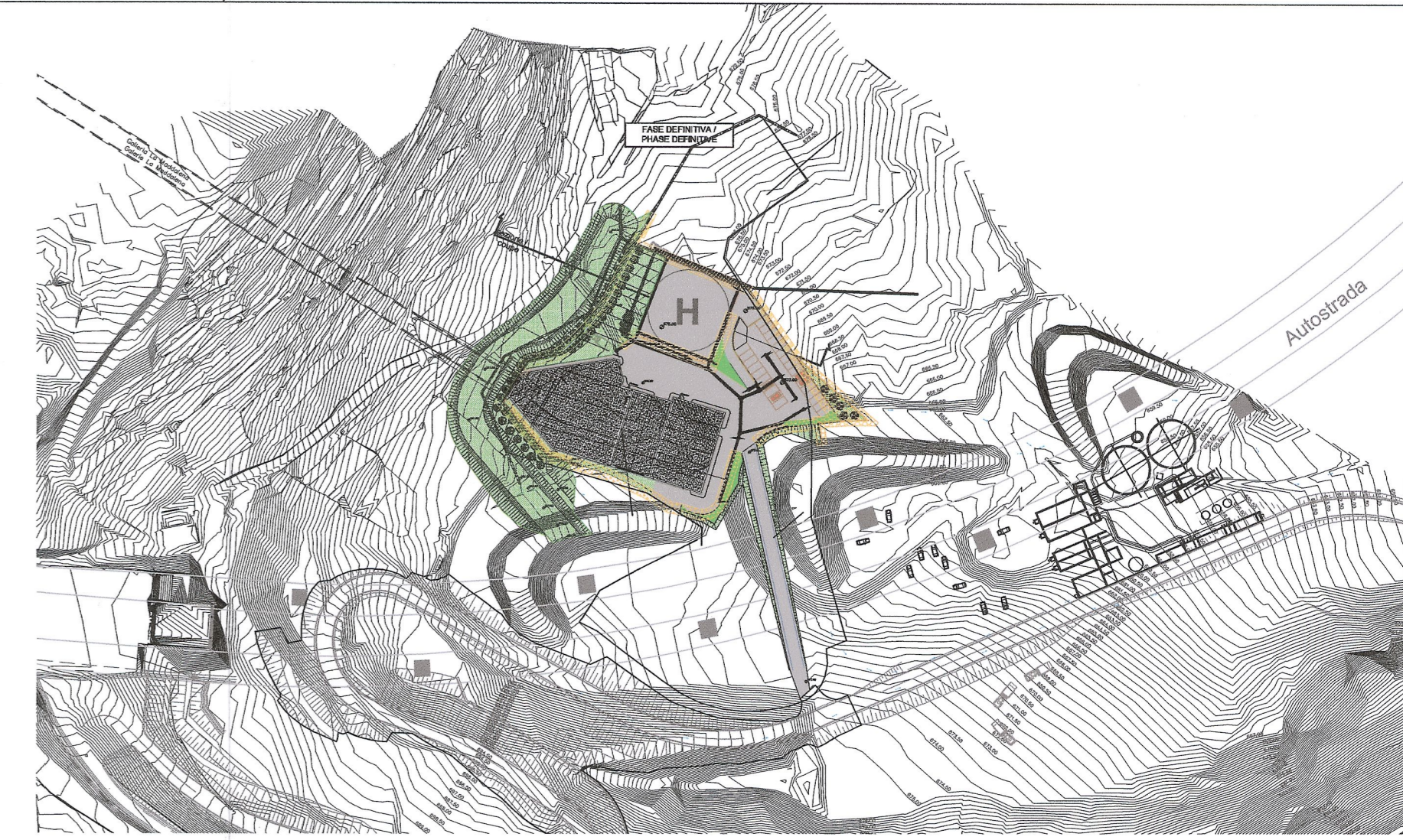
PLANIMETRIA - SCALA 1:2000 VUE EN PLAN - ECHELLE 1:2000
