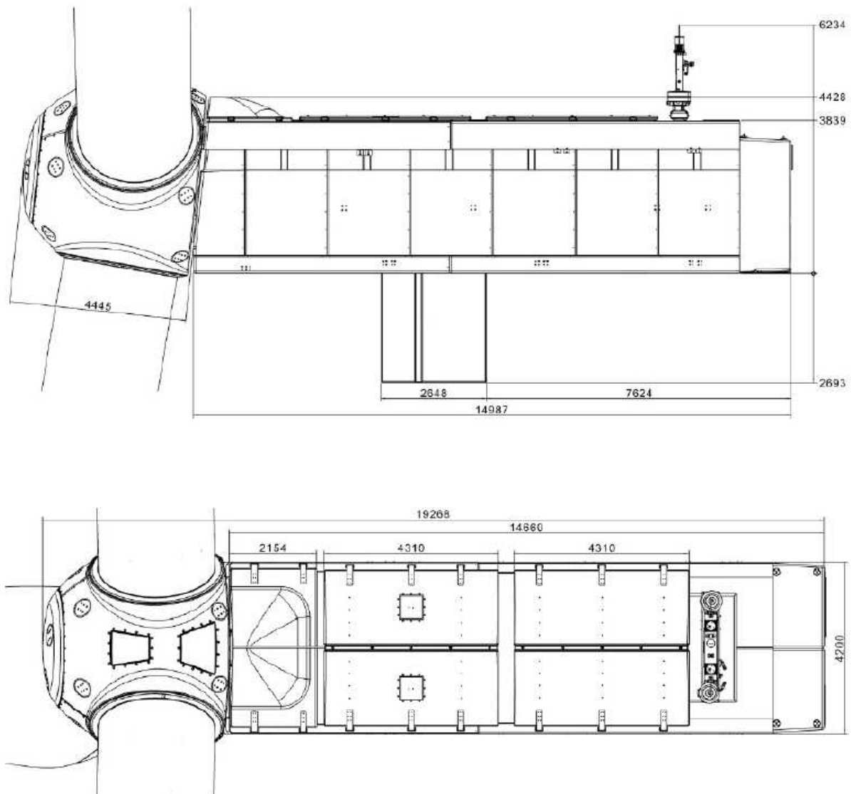
Figura c-2: Tipico navicella RIN16
