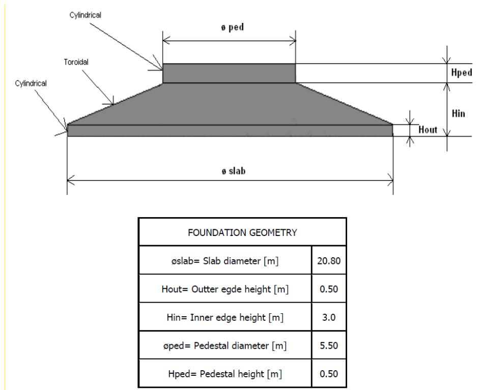
Figura d-1: Sezione tipo del plinto fondazione
