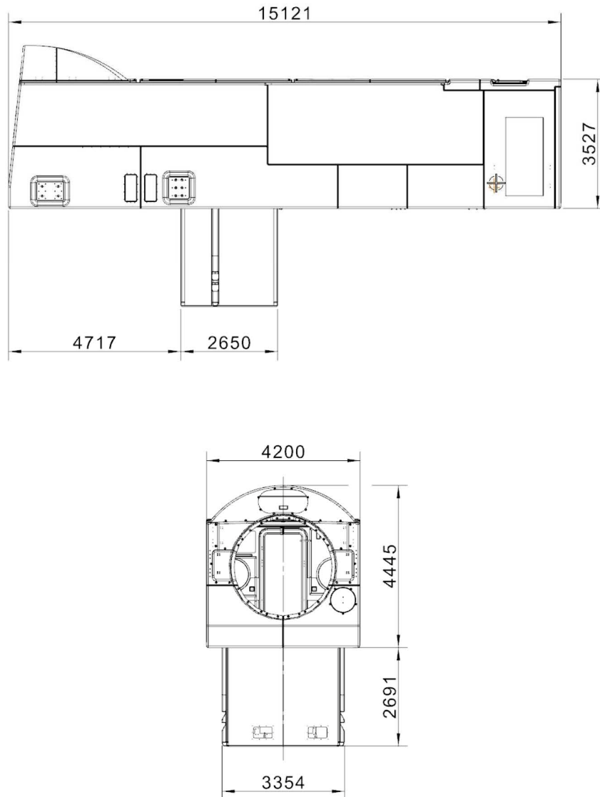
Figura c-3: Tipico navicella da RIN1 a RIN15 e RIN17
