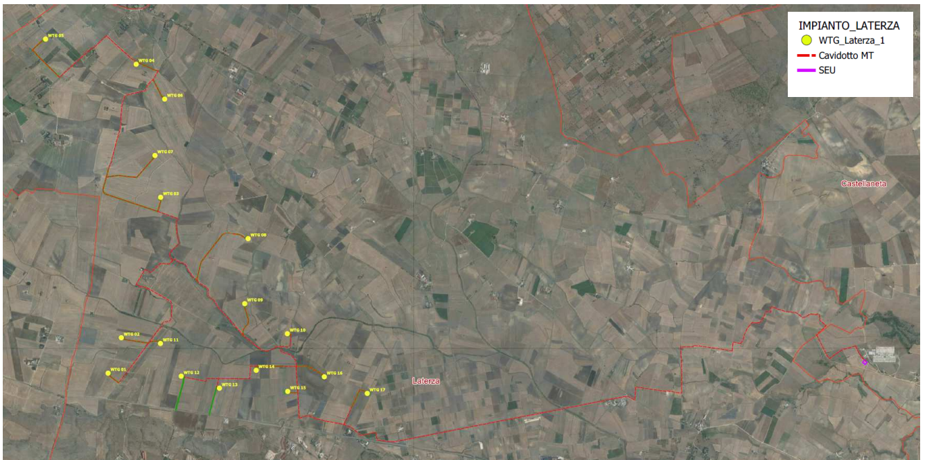
Figura 4-5: Area di intervento: dettaglio layout di progetto su ortofoto
