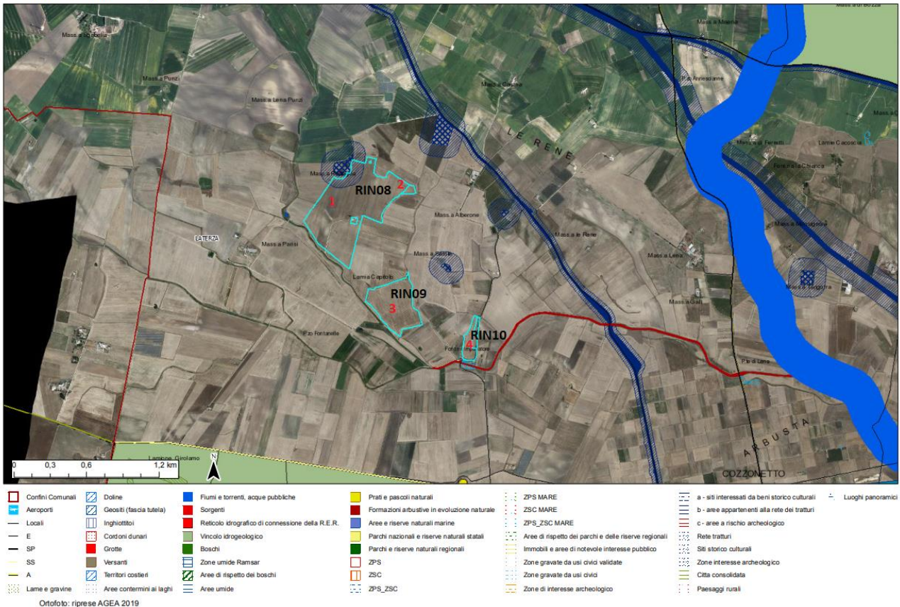
Figura 7-8: Punti cattura foto turbine RIN08-RIN09-RIN10
