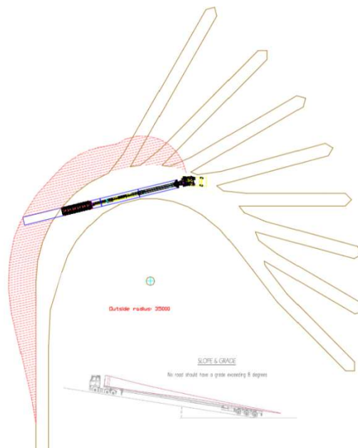
Figura 4 - Raggi minimi di curvatura ed ingombri da assicurare per il transito dei mezzi eccezionali sulla viabilità esterna al parco
