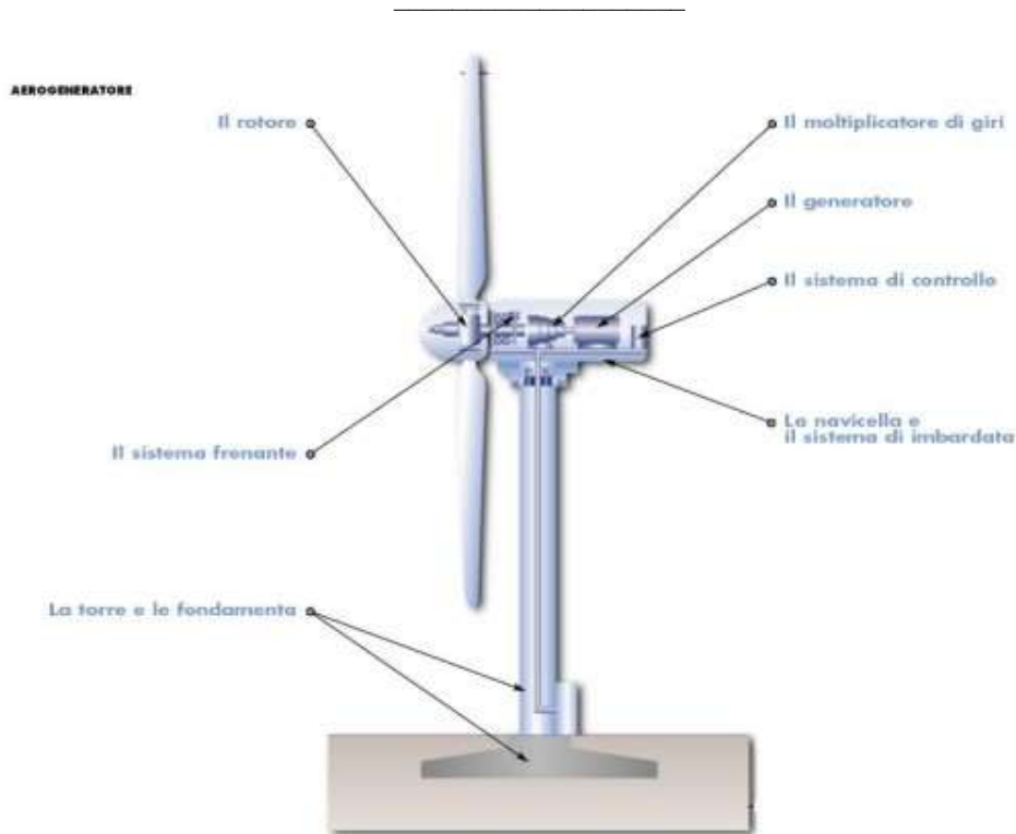
Figura 1 – Schematizzazione aerogeneratore
