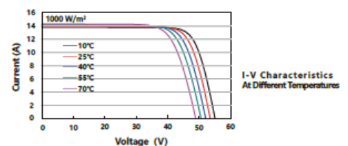
Figura 1 - Vista posteriore pannello, particolare struttura supporto, curva I-V del modulo di progetto.
