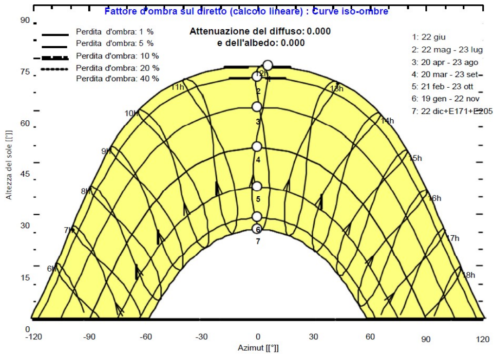
DIAGRAMMA ISO-OMBRE
