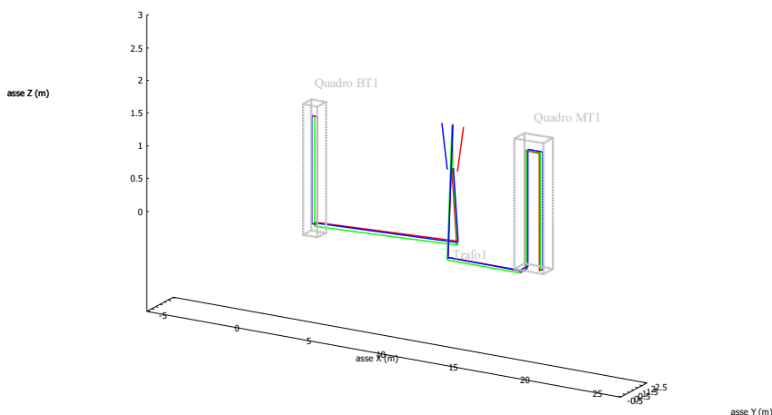
Modello spaziale cablaggi nelle cabine di trasformazione MT/BT
