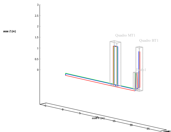
Modello spaziale cablaggi nelle cabine di ricezione
