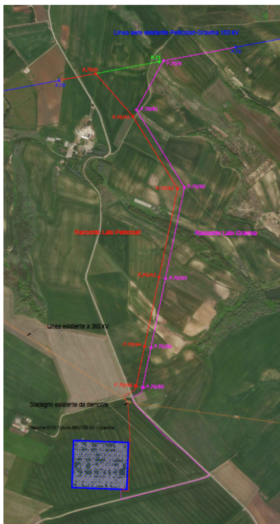
Figura 1: Inquadramento delle opere su Ortofoto della futura SE “Altamura 36 kV” e dei raccordi 150kV alla linea “Pellicciari-Gravina-Altamura”
