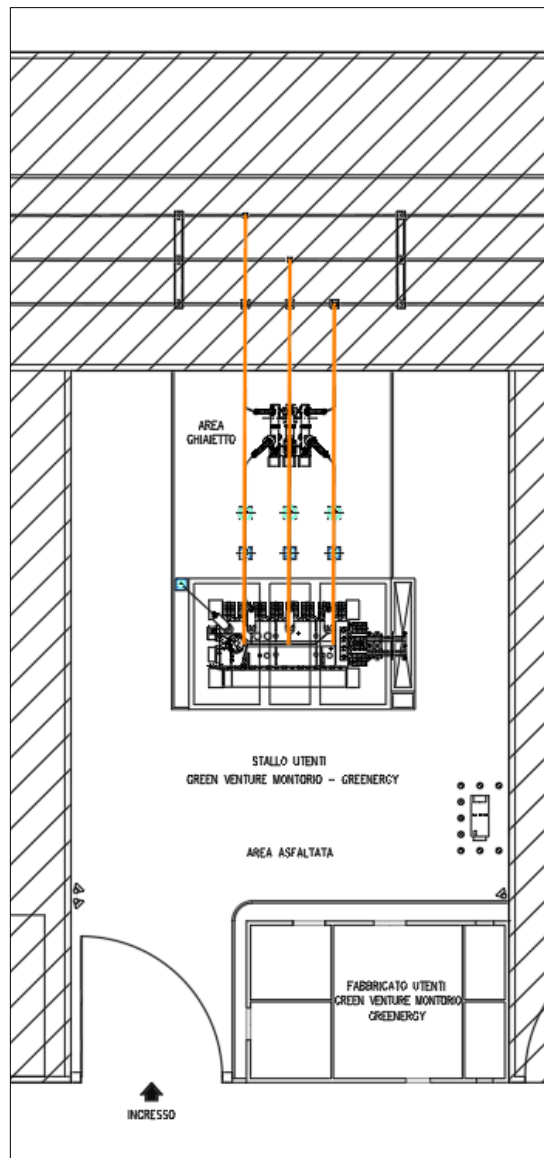
Figura 3 – Planimetria della cabina utente con individuazione degli elementi attivi
