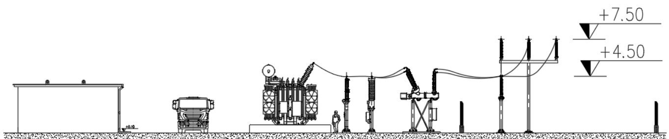
Figura 2 – Sezione della cabina utente e Sbarra AT comune con individuazione delle altezze
