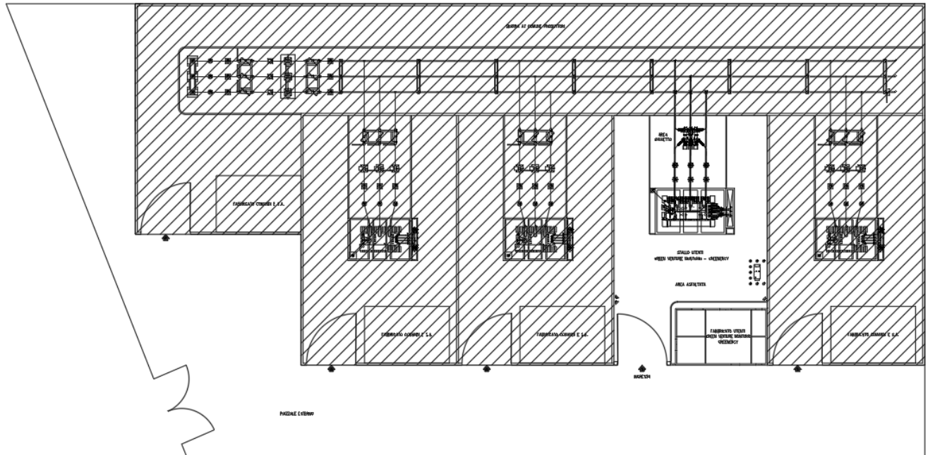
Figura 1 – Planimetria della cabina utente (senza retino), all'interno del Punto di Raccolta (con retino)
