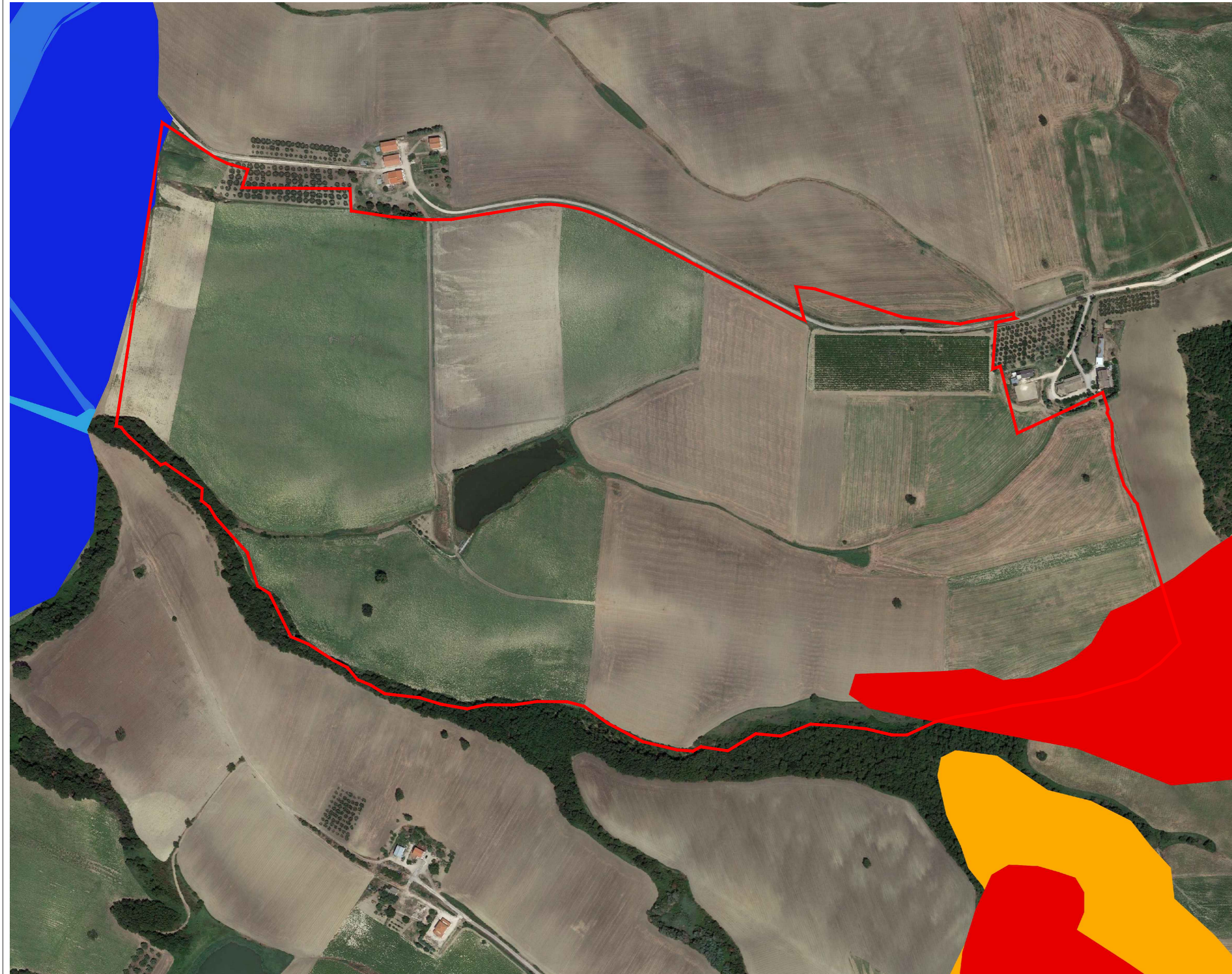
STRALCIO CARTA IDROGEOMORFOLOGICA SCALA 1:5000
