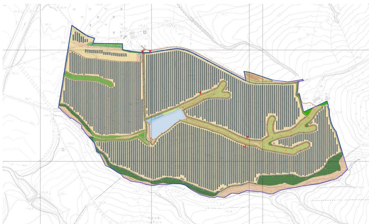
Figura 34: Layout di impianto su base CTR con le aree destinate a progetto agricolo
