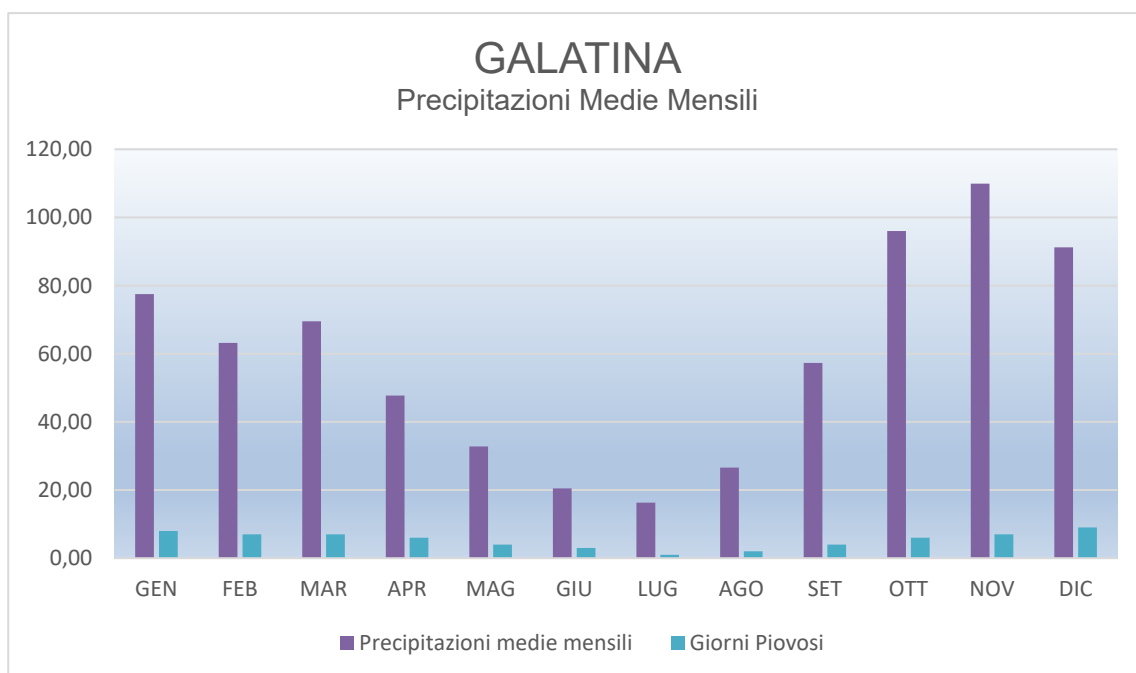
Figura 5.3 – Precipitazioni medie mensili e numero dei giorni piovosi nella stazione pluviometrica di Galatina - Anno idrologico medio 1921 - 2020.
