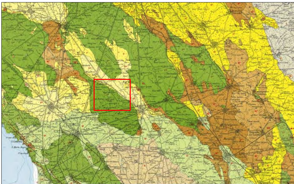
Figura 3.1: Estratto della Carta Geologica d'Italia in scala 1:100000 – Foglio 204 (Gallipoli).
