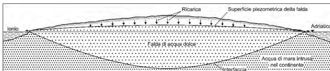
Figura 6.2: Sezione idrogeologica schematica della Penisola Salentina. La falda
