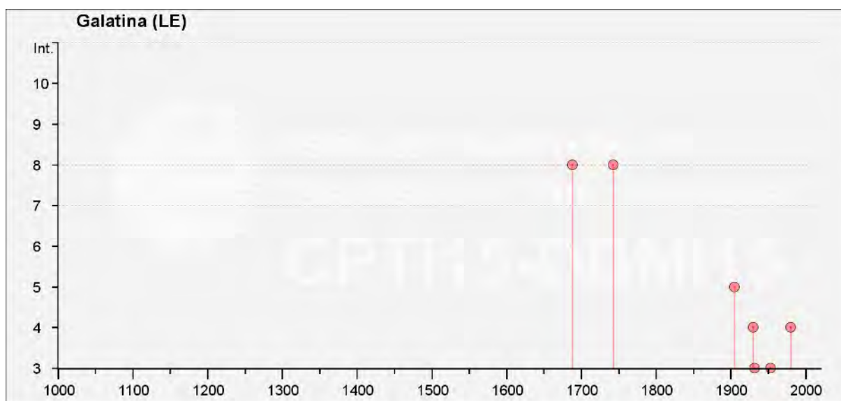
Figura 7.3 – Storia sismica del Comune di Galatina [40.175, 18.168] – https://emidius.mi.ingv.it/CPTI15-DBMI15_v1.5/query_place/
