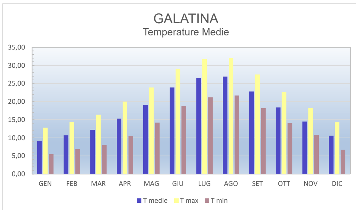
Figura 5.2: Andamento delle temperature medie mensili registrate nella stazione di Galatina
