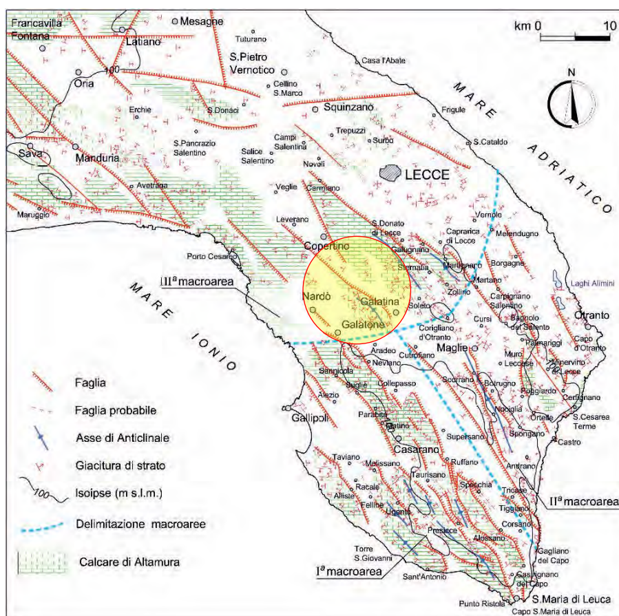
Figura 2.2: Carta tettonica della Penisola Salentina.
