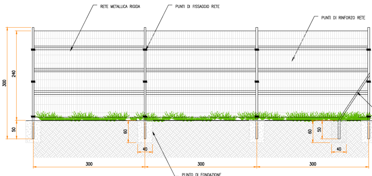
Figura 4.5: Tipica recinzione
