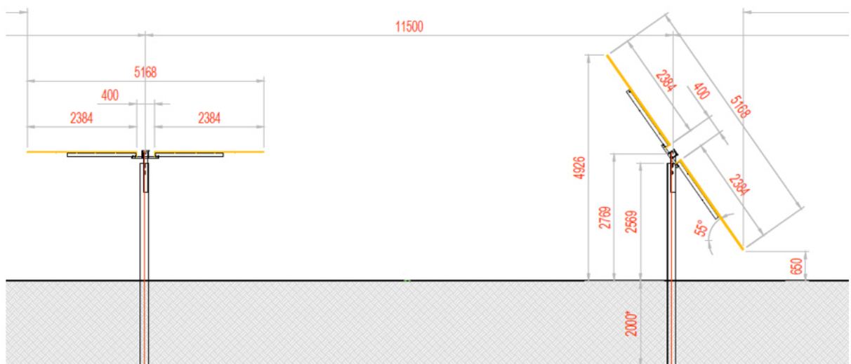
Figura 4.2: Particolare strutture di sostegno moduli
