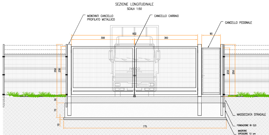
Figura 4.6: Tipo cancello
