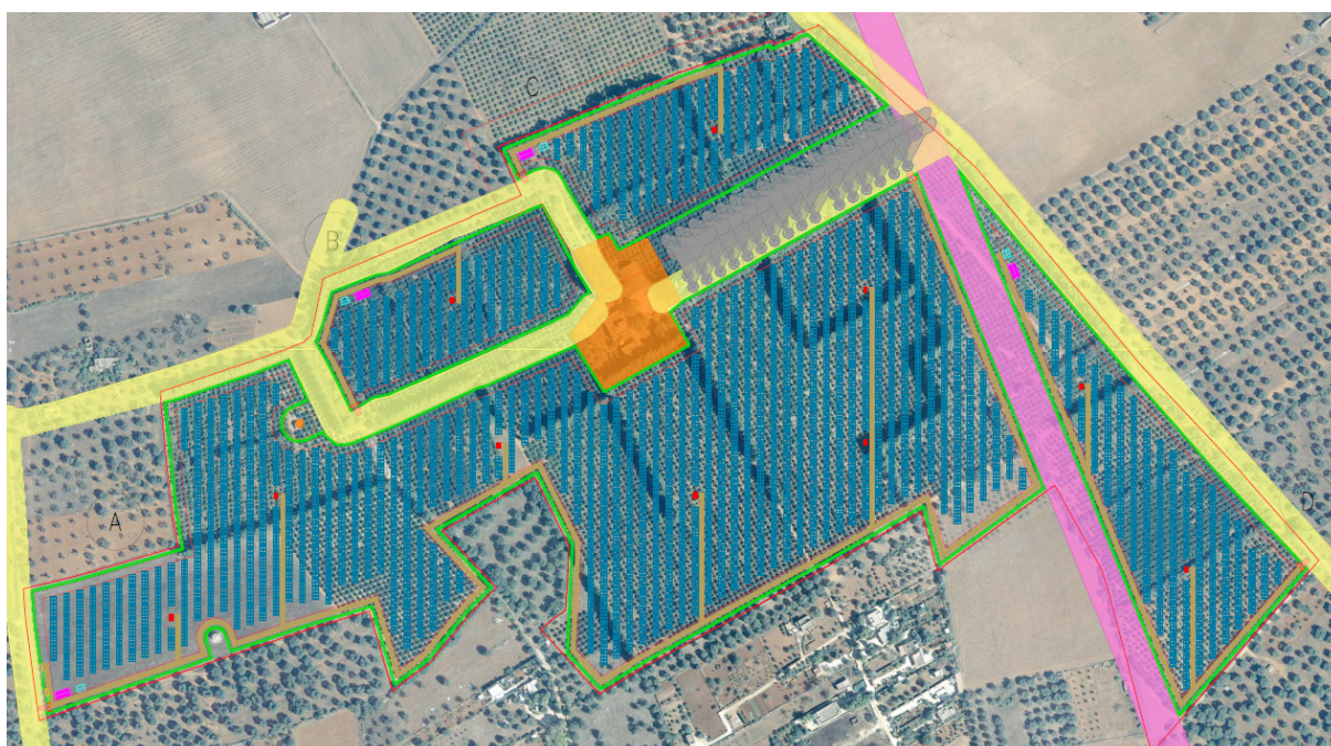
Figura 2.3: Layout di progetto
