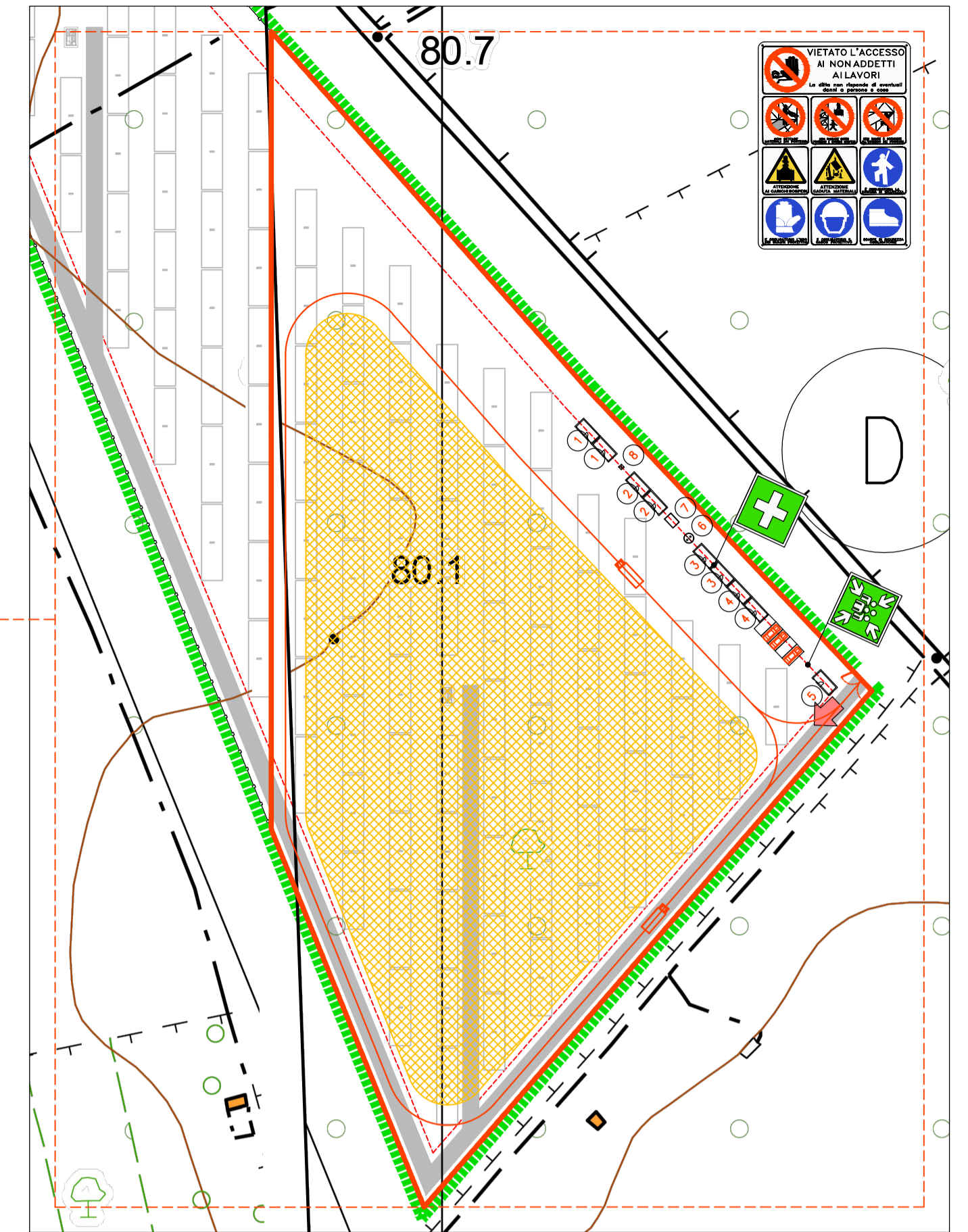
DETTAGLIO CARTOGRAFICO AREA D - SCALA 1:1250 SCALA 1:1250 - 1 cm = 12.5 m
