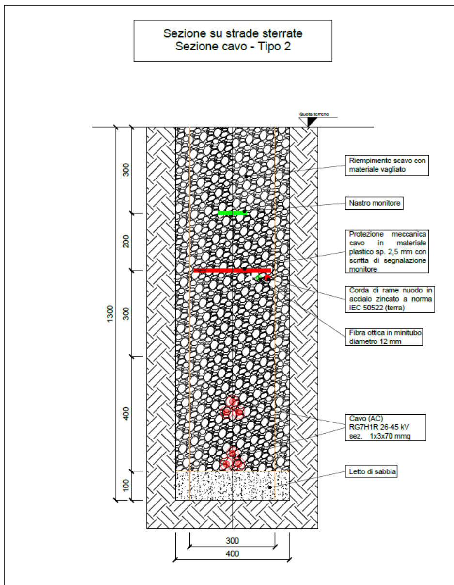
Fig. 6.5.6-2 Tipico sezione di posa con due circuiti interni
