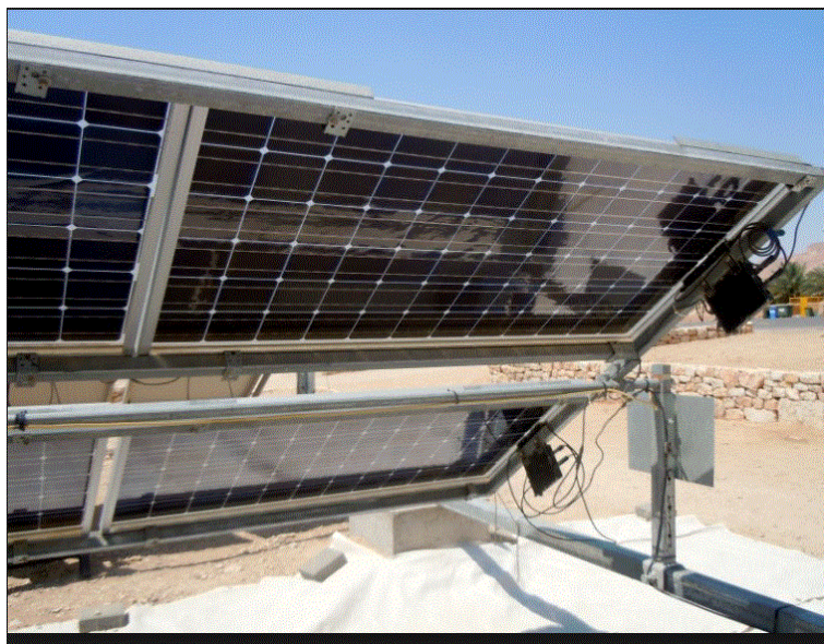
Fig. 5.1-1 Tipico Modulo fotovoltaico Bifacciale
