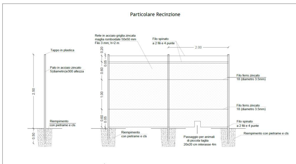
fig. 9.1.8-1- Recinzione esterna
