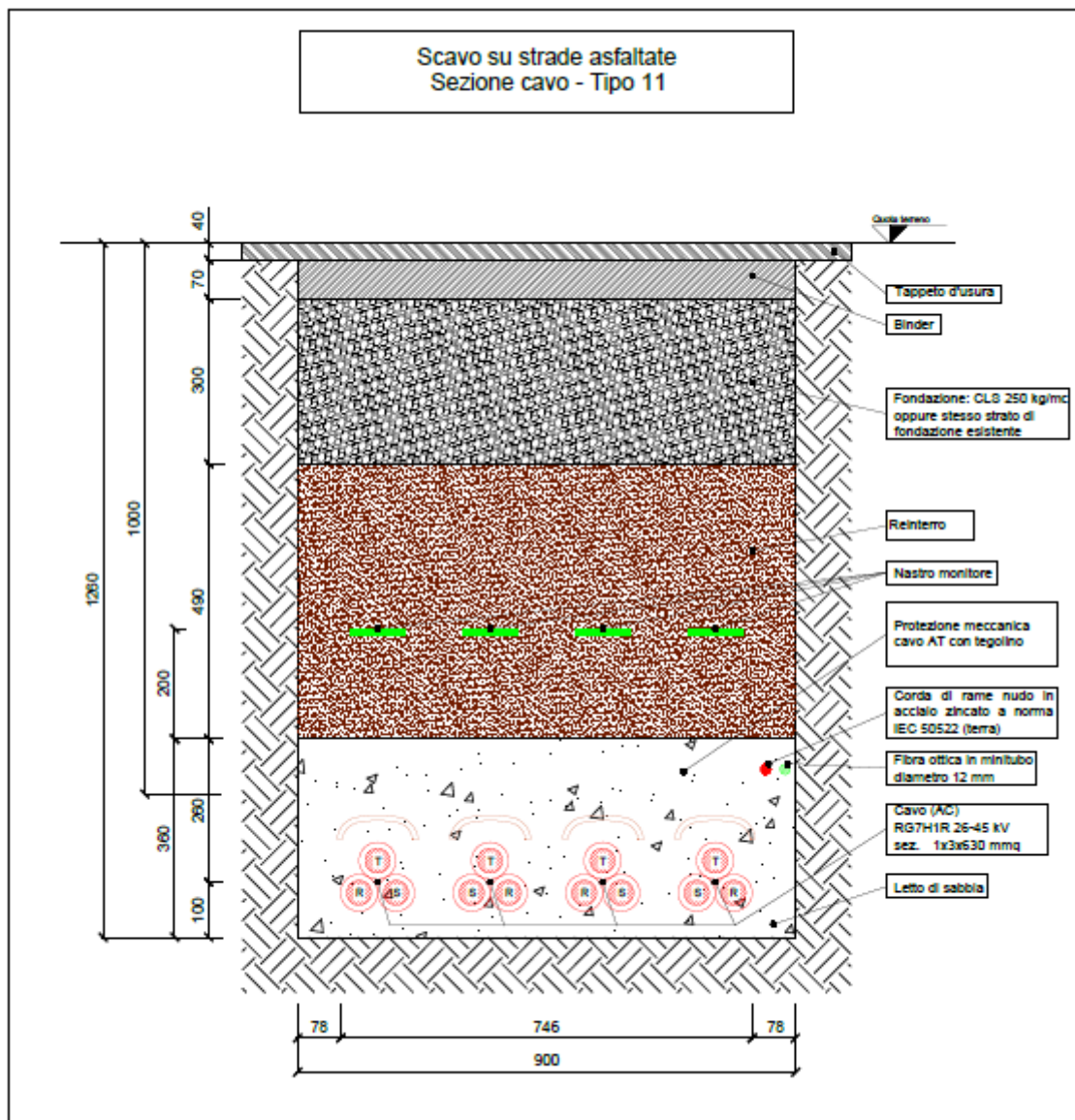
Fig. 6.5.6-7 Tipico sezione di posa dorsale di connessione con quattro cavidotti
