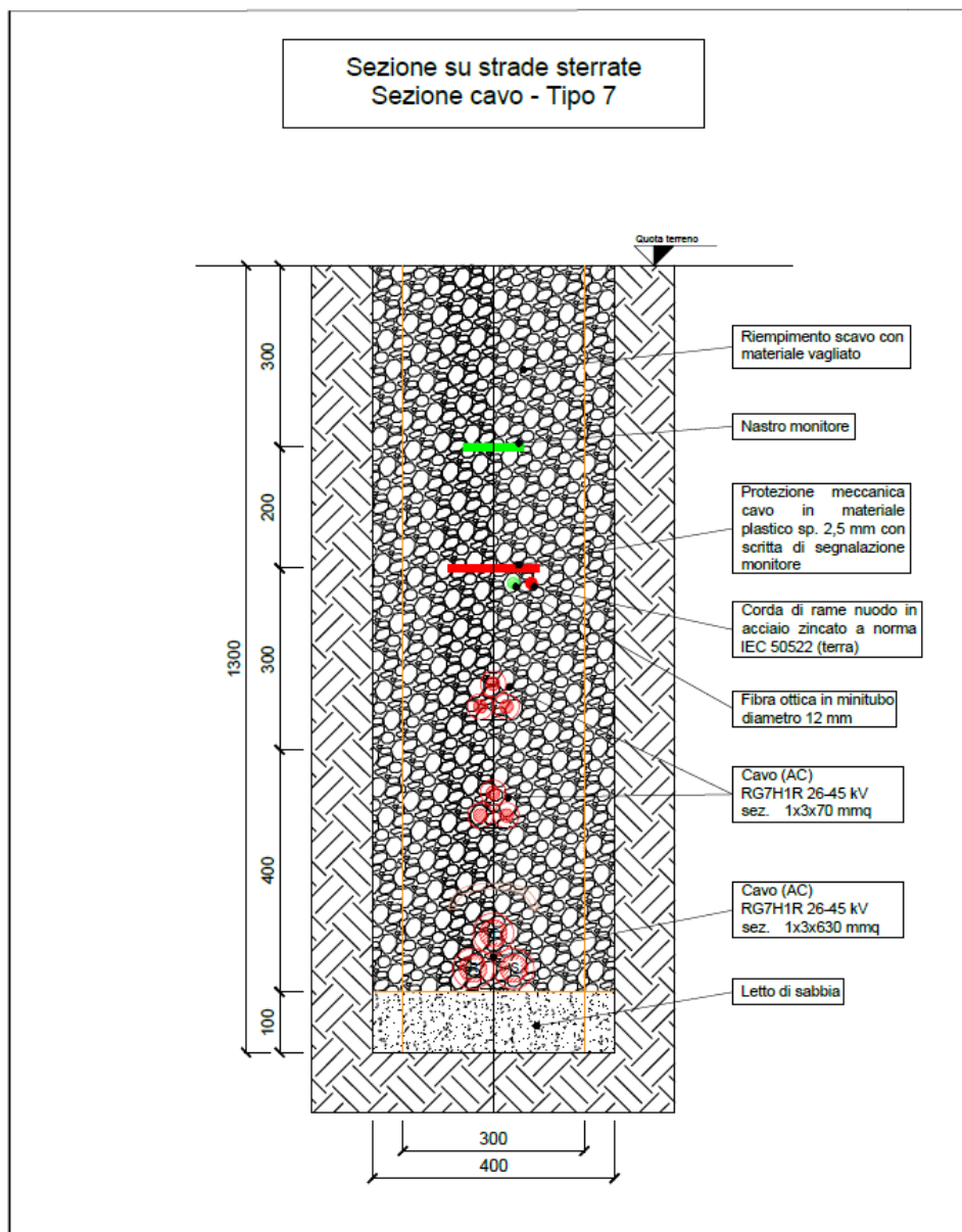
Fig. 6.5.6-3 Tipico sezione di posa con tre cavidotti
