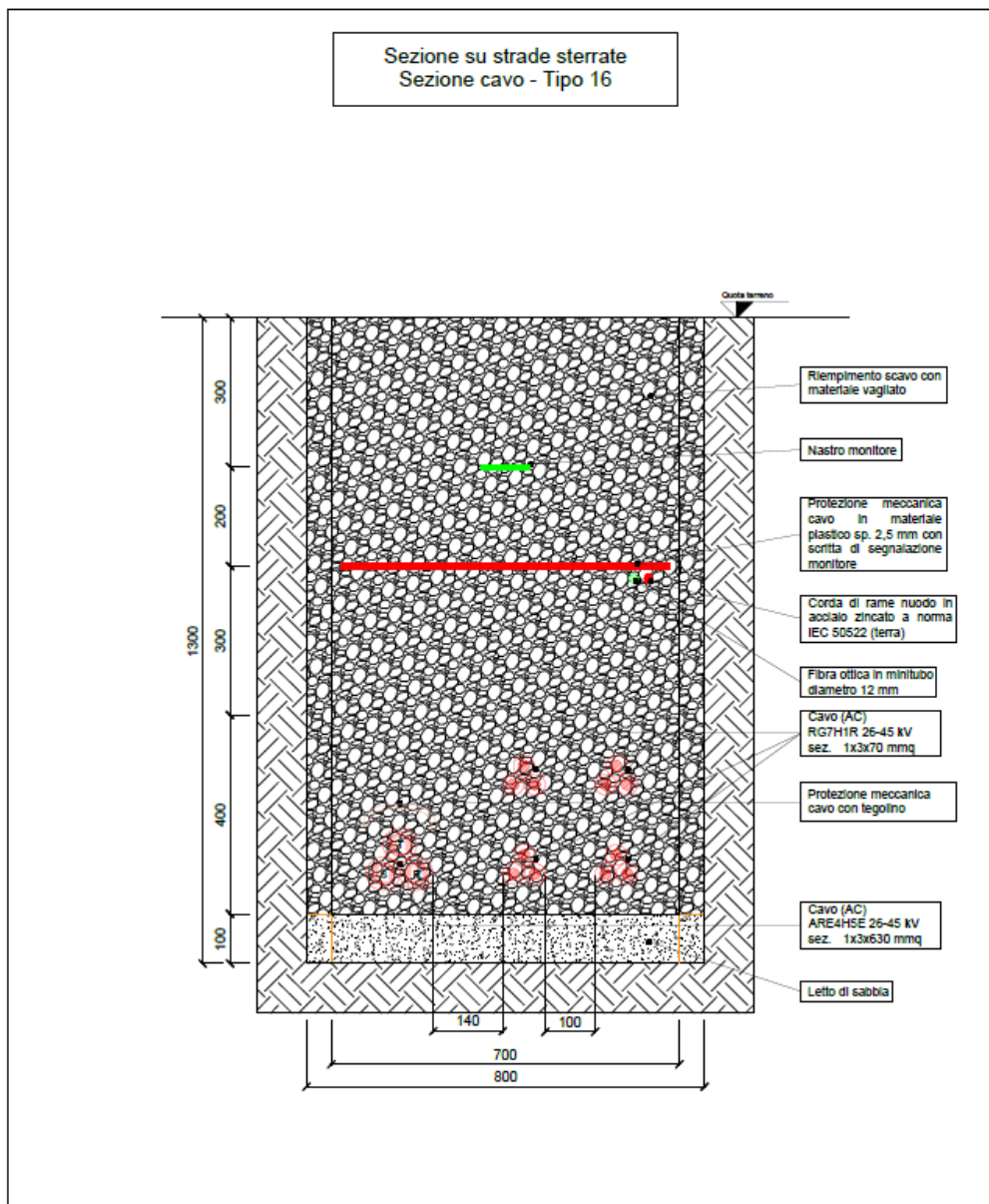
Fig. 6.5.6-4 Tipico sezione di posa con quattro cavidotti
