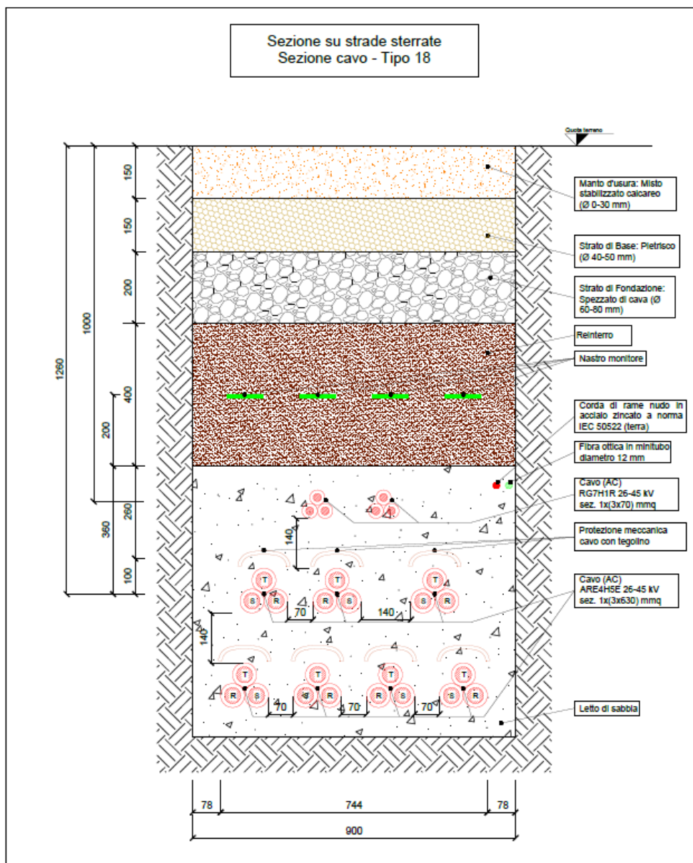
Fig. 6.5.6-6 Tipico sezione di posa con nove cavidotti
