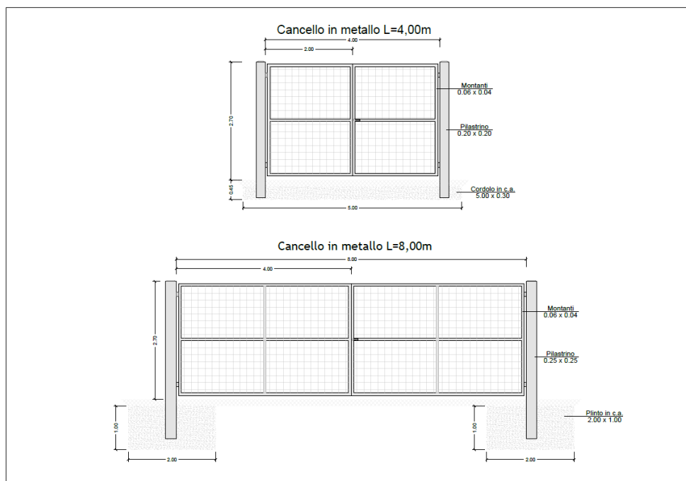
fig. 9.1.8-1- Cancelli d'ingresso
