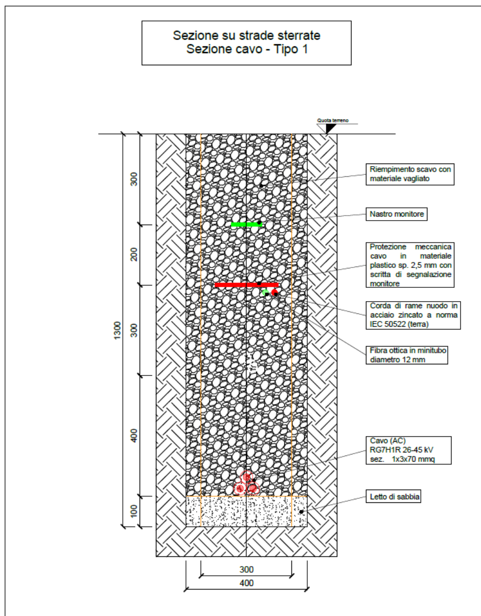
Fig. 6.5.6-1 Tipico sezione di posa con un cavidotto interno
