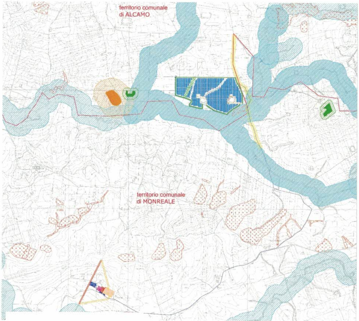
Fig. 3. Integrazioni volontarie 08/11/2022 – Opere in progetto su carta dei vincoli
