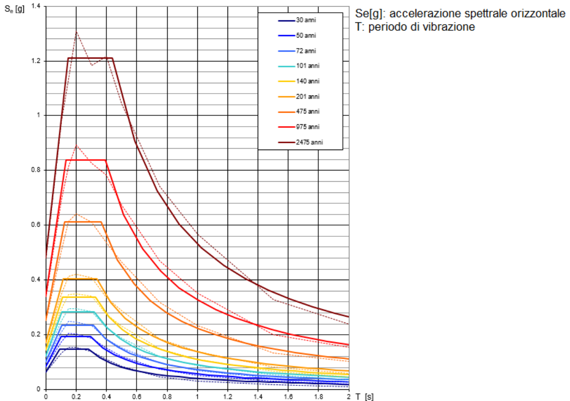
Figura 3.1 – Spettri di risposta elastici per periodi di ritorno T_r di riferimento (le linee continue rappresentano gli spettri di Normativa, le linee tratteggiate si riferiscono a agli spettri di progetto S1-INGV da cui sono derivati).
