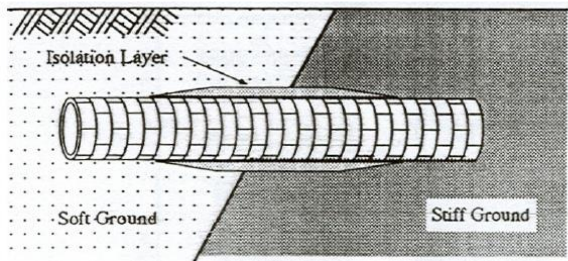
Figura 4.3 – Isolamento esteso del tunnel (Kawashima, 2000)
