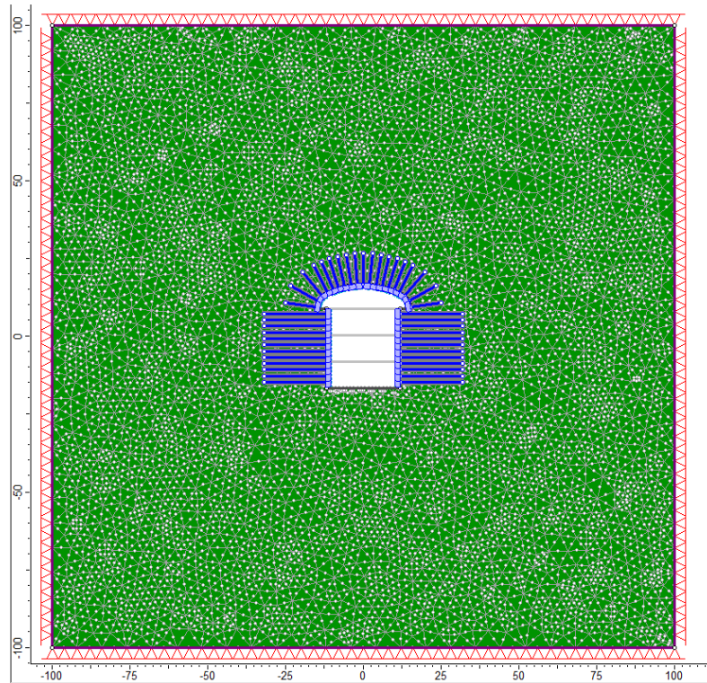
Figura 4.1 – Centrale in caverna: Geometria del modello numerico per le analisi statiche relativa all'ultimo step della simulazione
