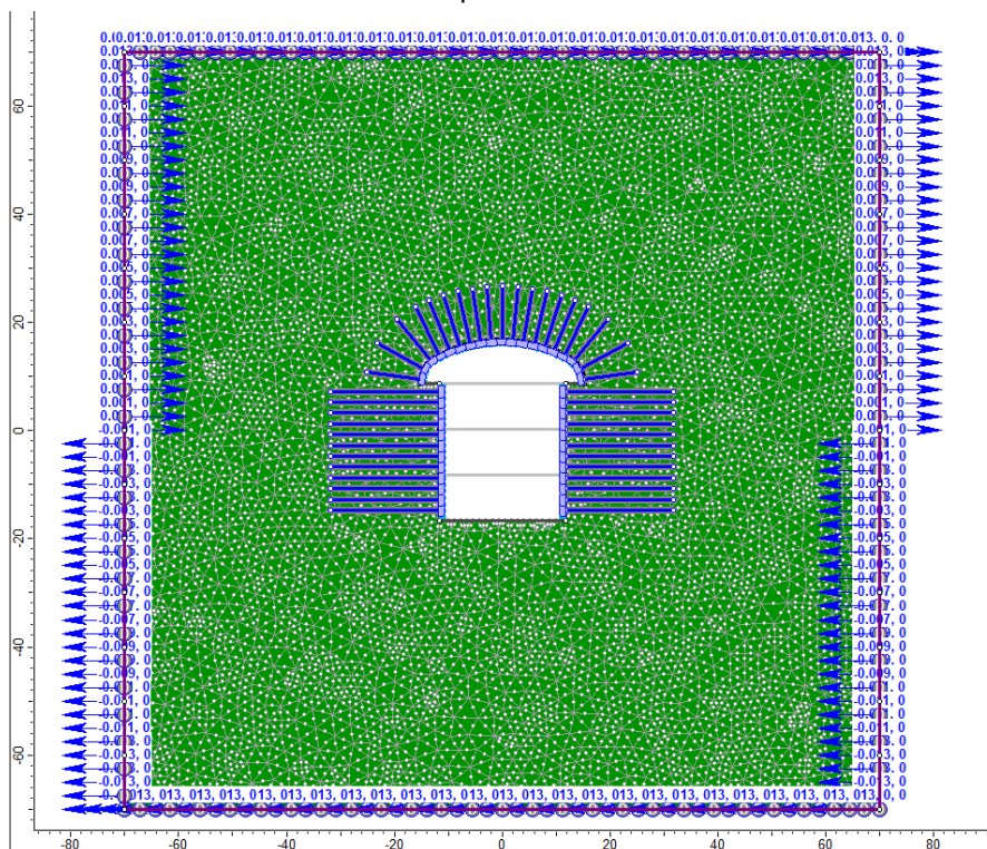
Figura 4.2 – Centrale in caverna: Geometria del modello numerico per le analisi sismiche relativa all'ultimo step della simulazione
