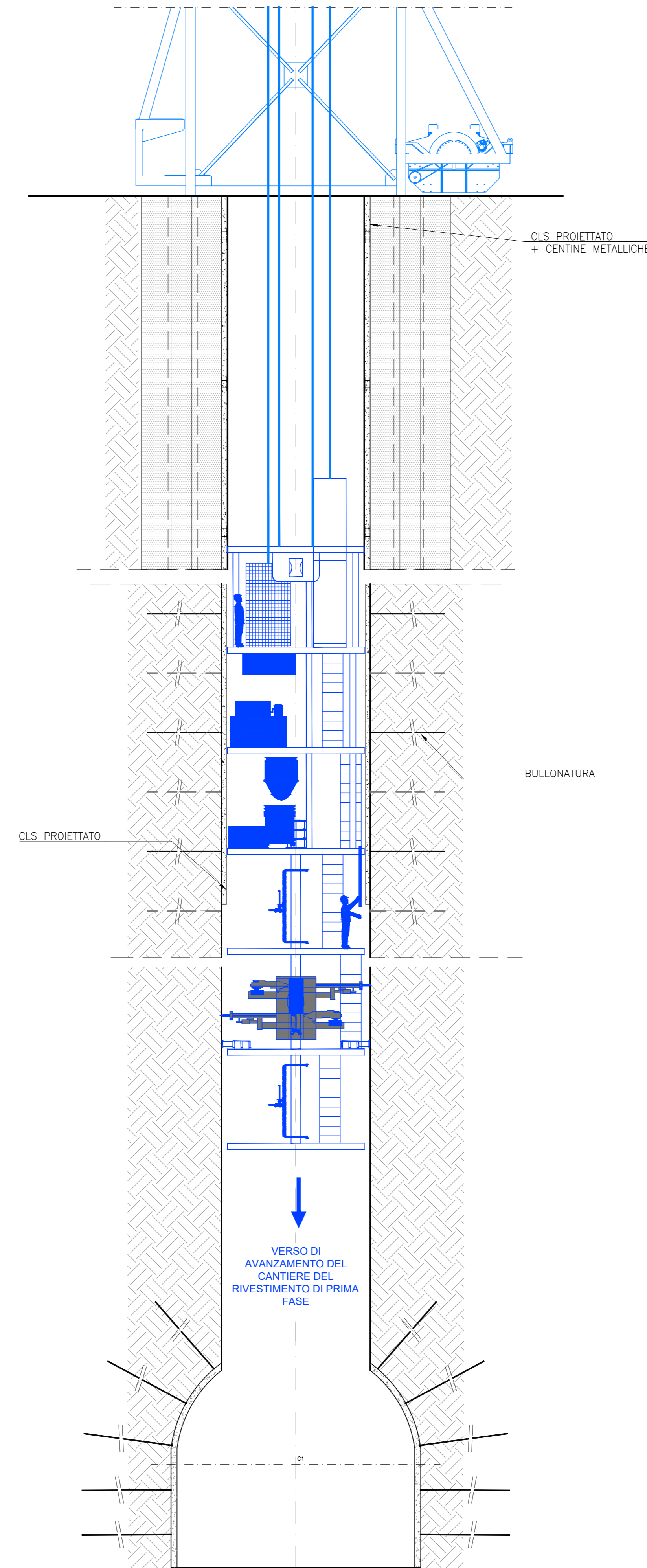
FASE 3: MESSA IN OPERA INTERVENTI DI SOSTEGNO DI PRIMA FASE
