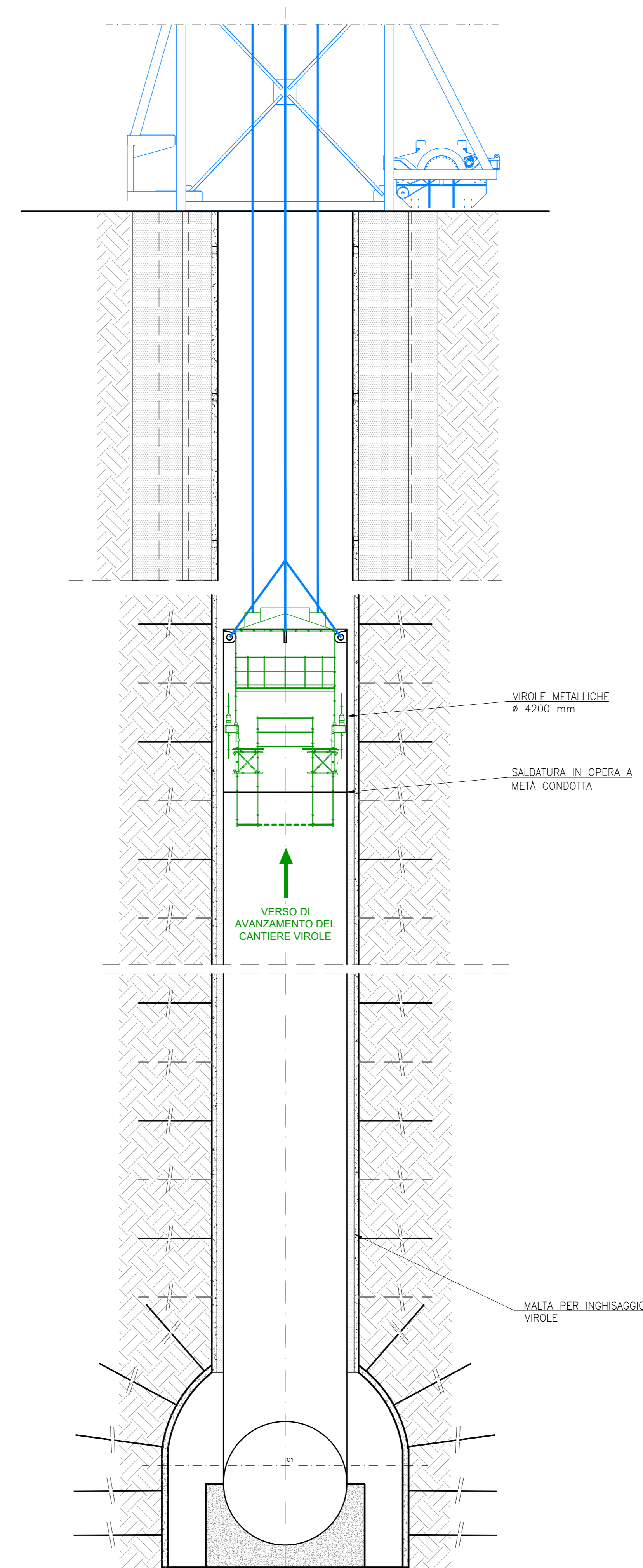
FASE 4: INGHISAGGIO VIROLE METALLICHE
