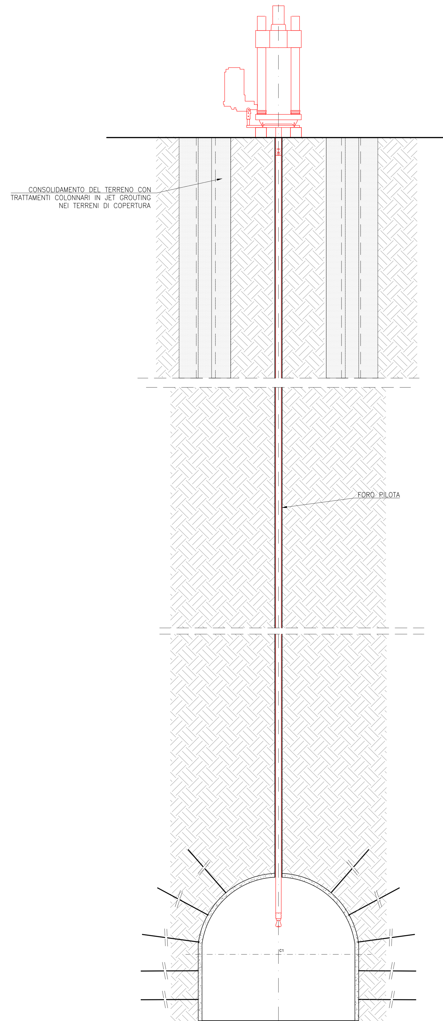
FASE 1: ESECUZIONE DEL FORO PILOTA
