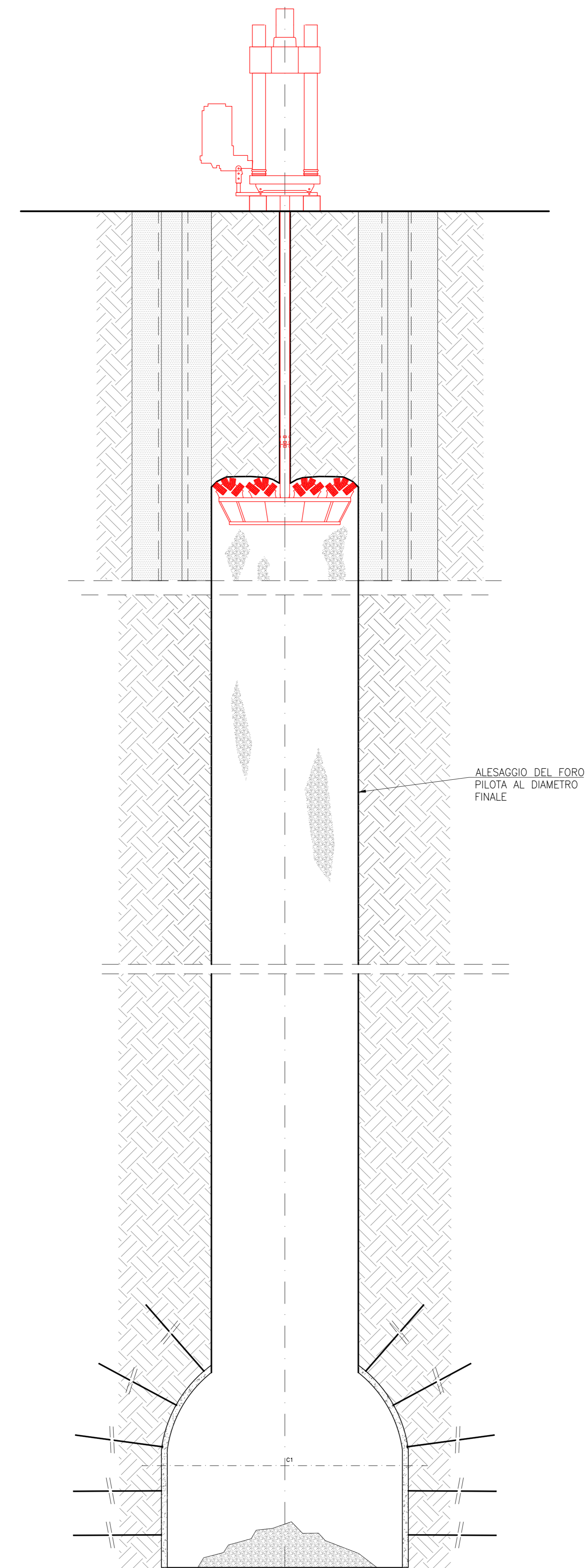
FASE 2: ALESAGGIO DEL FORO PILOTA
