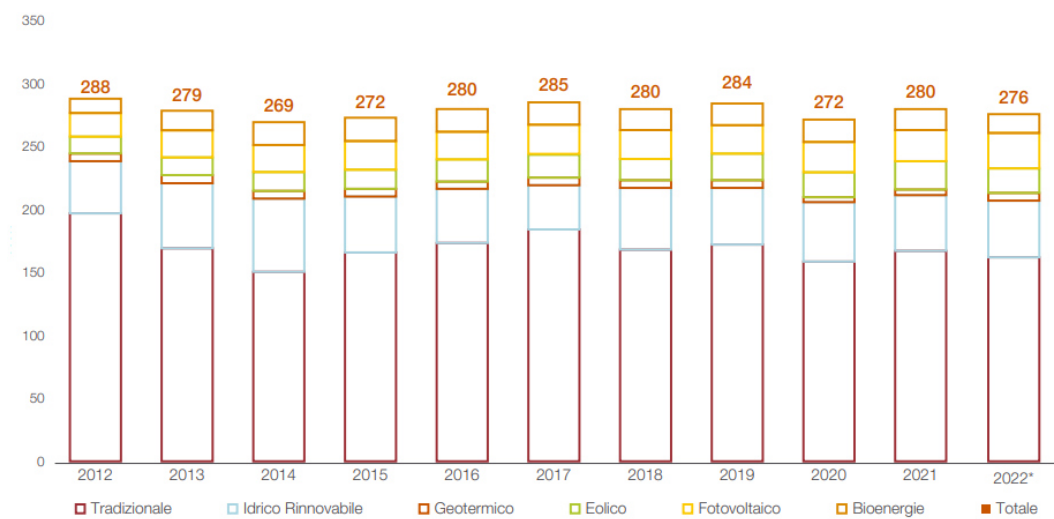
Evoluzione produzione netta nazionale per fonte (TWh)
