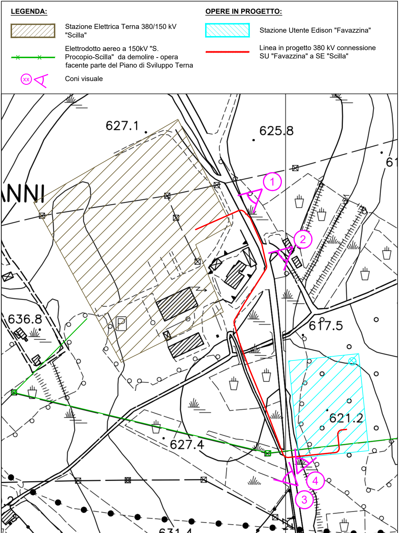
Planimetria coni visuale
