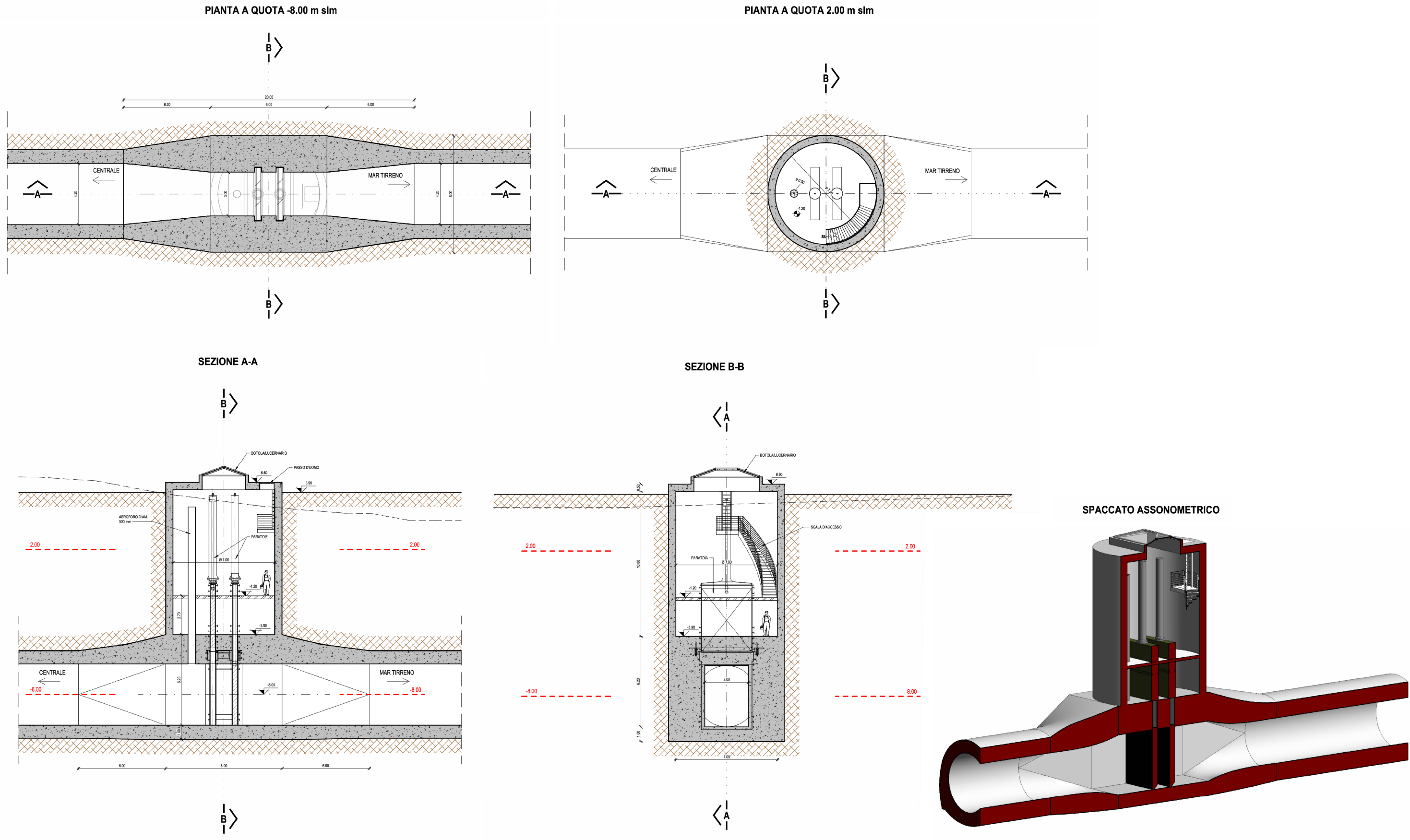
FIGURA 4.3 POZZO PARATOIE PIANTE E SEZIONI
