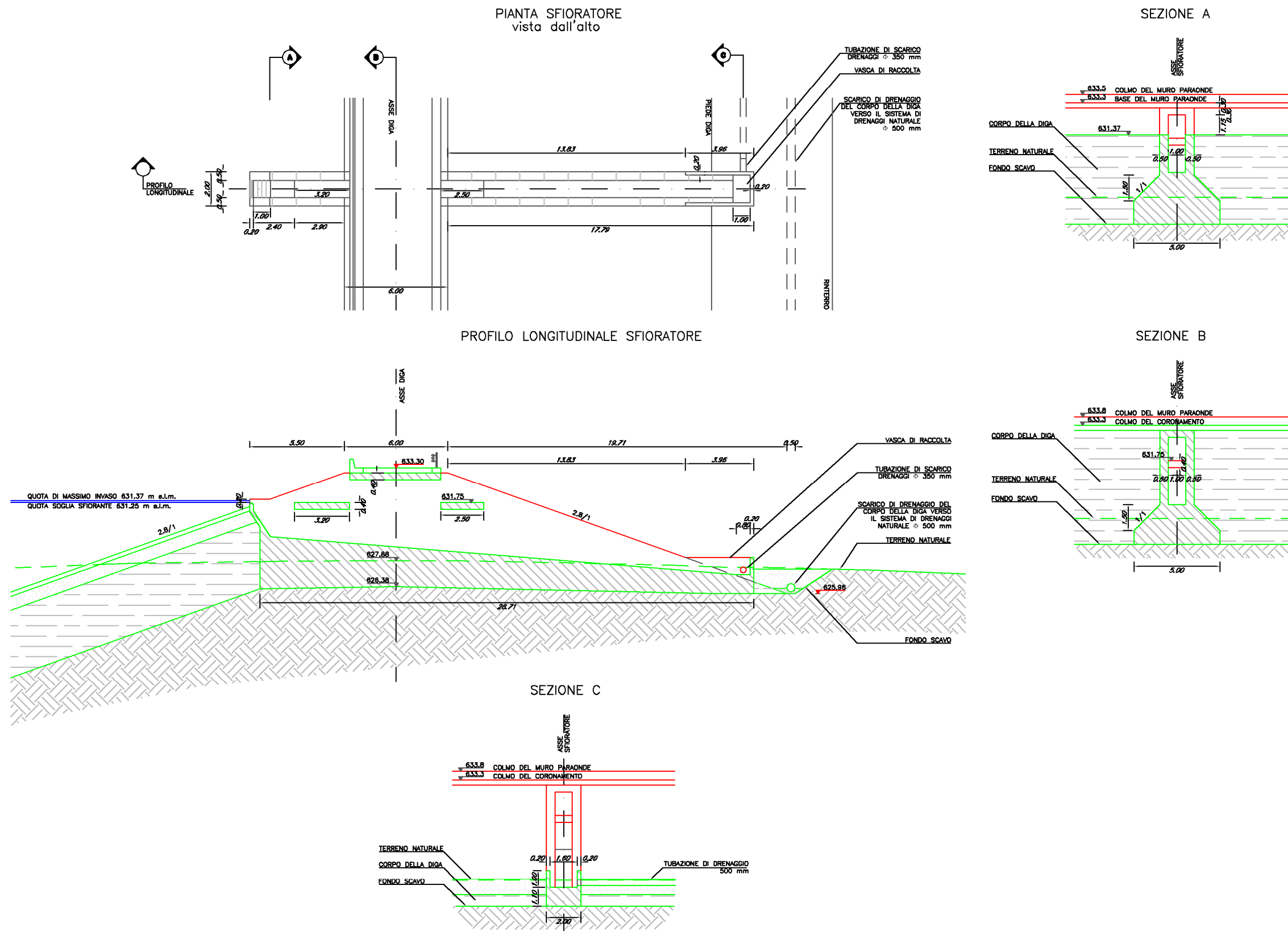
SFIORATORE DI SUPERFICIE E CANALE DI DRENAGGIO – TIPOLOGICO, PROFILI E SEZIONI
