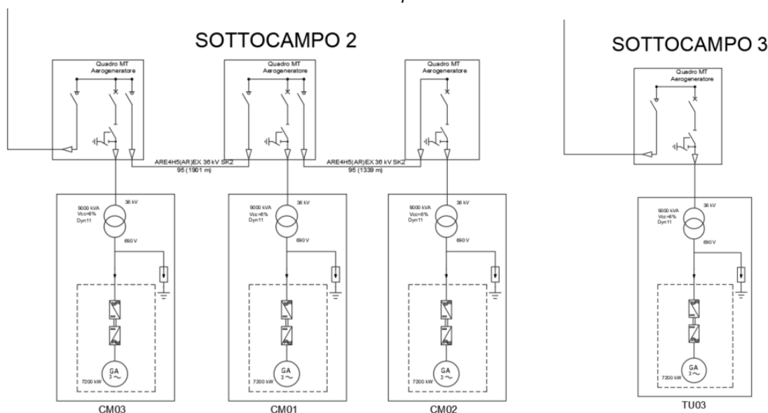
Schema a blocchi del parco eolico GRUPPO 2 E GRUPPO 3
