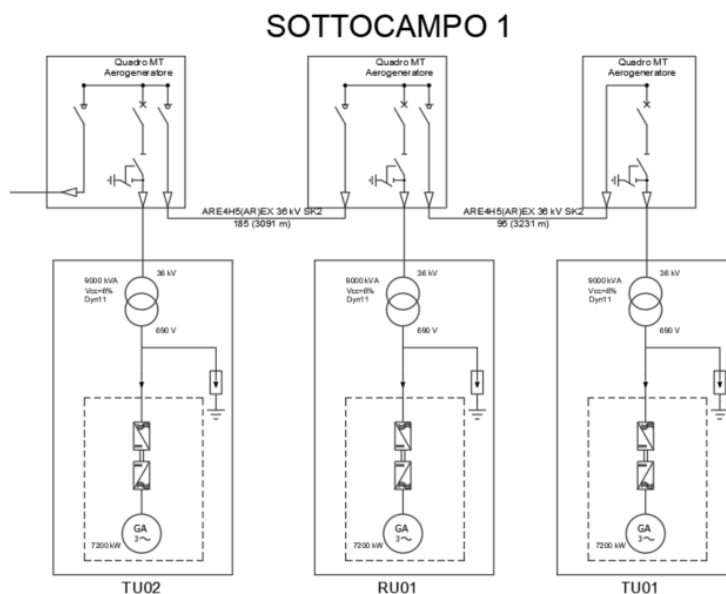
Schema a blocchi del parco eolico GRUPPO 1
