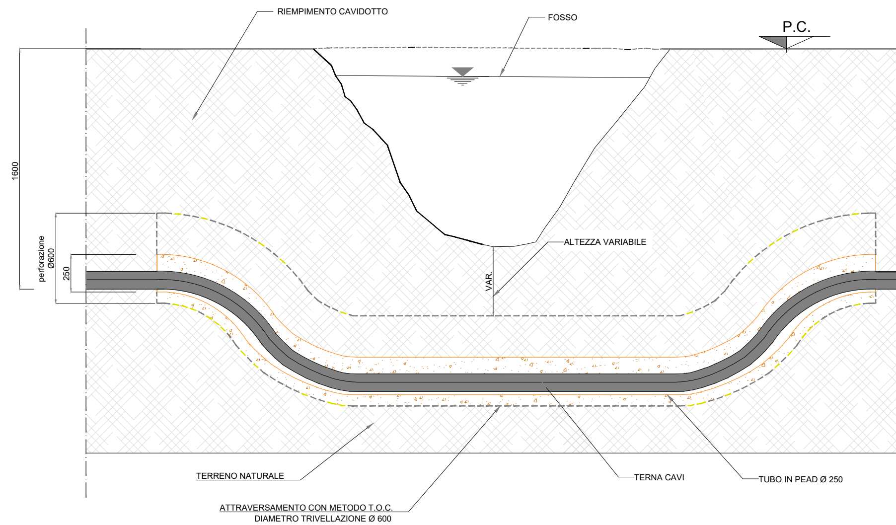
SEZIONE LONGITUDINALE
