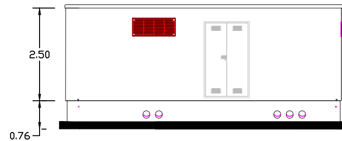
PROSPETTO CABINE
