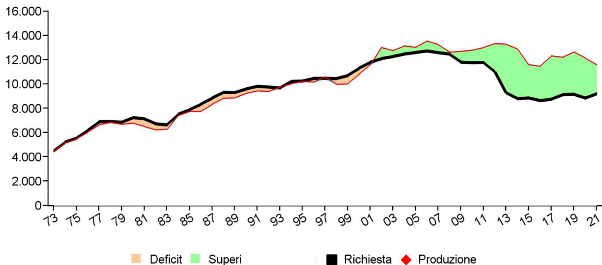
Dati TERNA 2021 - produzione energia elettrica Sardegna
