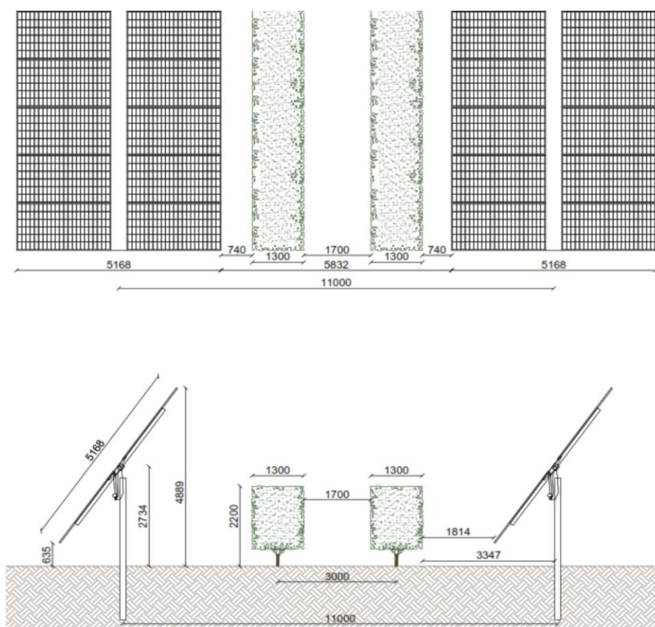
Figura 12. Dettaglio layout impianto agri-voltaico
