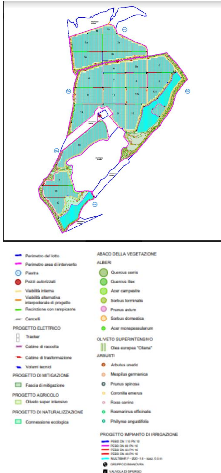
Figura 11. Dettaglio layout impianto di irrigazione
