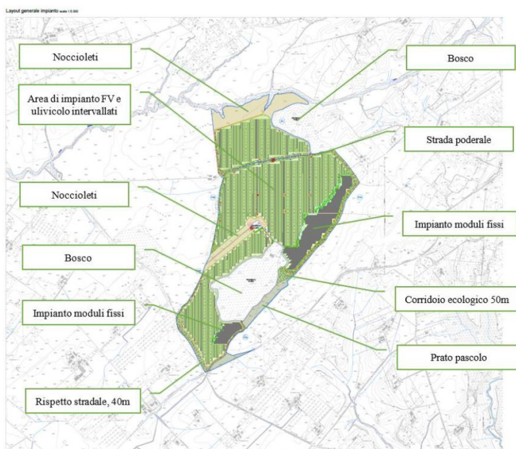
Figura 5 - Lay generale dell'impianto,
