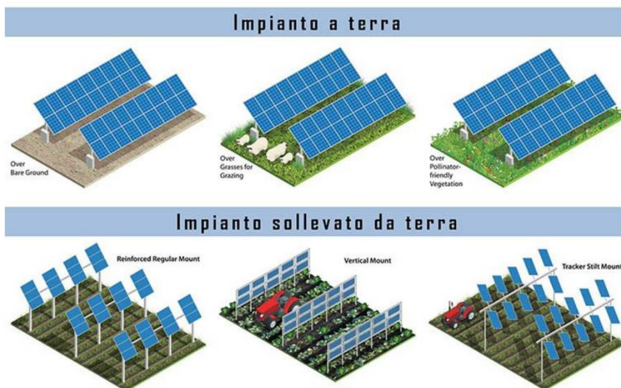
Figura 32 - Tipologie di impianti agrovoltai, fonte NREL
