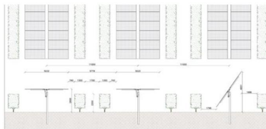
Figura 3 - Impostazione agrivoltaica
