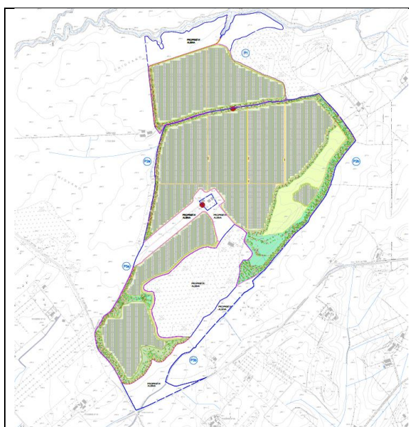
Figura 33- Veduta impianto
