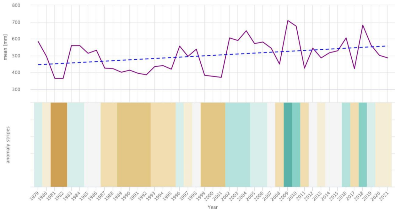
Figura 3. Stima delle precipitazioni totali medie annuali per Orta Nova e dintorni dal 1979 al 2021 (ERA5, ECMWF). La linea blu tratteggiata mostra la tendenza lineare del cambiamento climatico. In basso le strisce anomalia che rappresentano la precipitazione totale di un anno: verde per gli anni più umidi e marrone per quelli più secchi.
