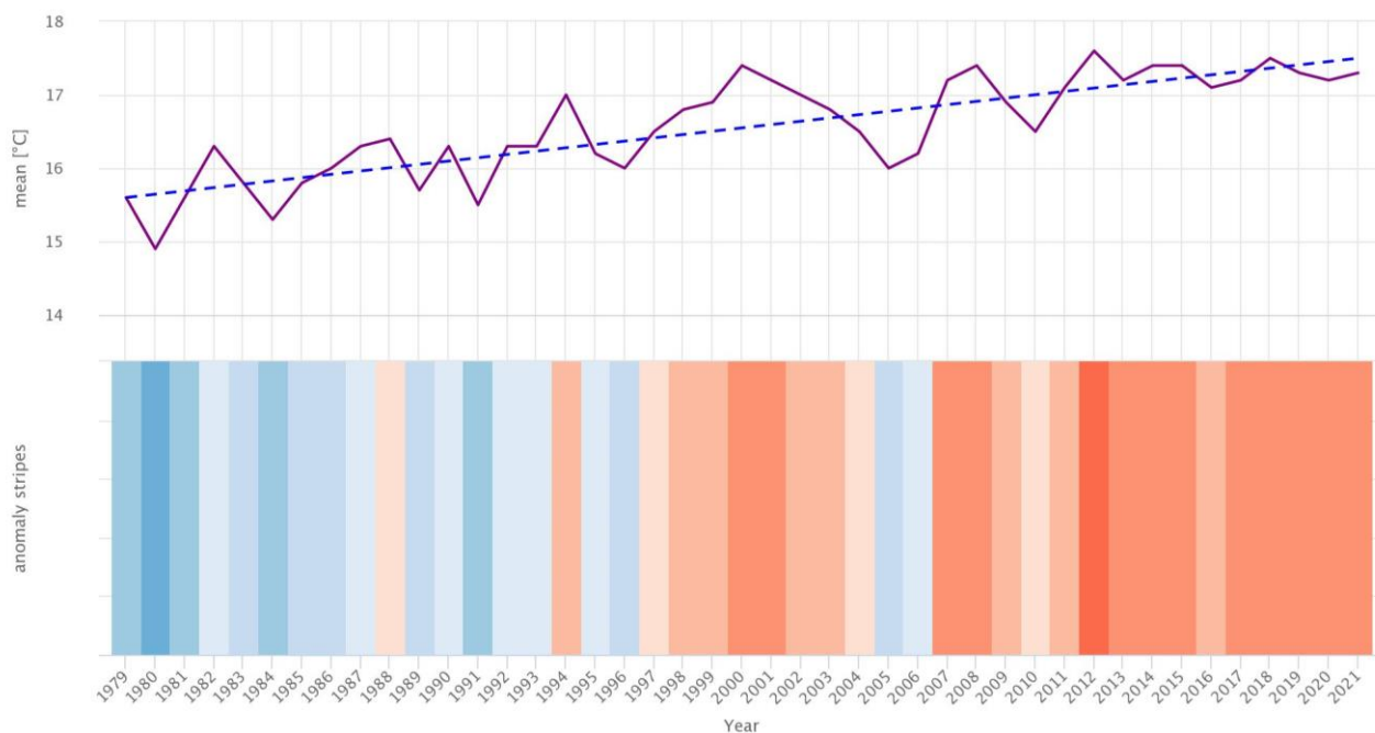
Figura 2. Stima della temperatura media annuale per Orta Nova e dintorni dal 1979 al 2021 (ERA5, ECMWF). La linea blu tratteggiata mostra la tendenza lineare del cambiamento climatico. In basso le strisce anomalia che rappresentano la temperatura media di un anno: blu per gli anni più freddi e rosso per quelli più caldi.
