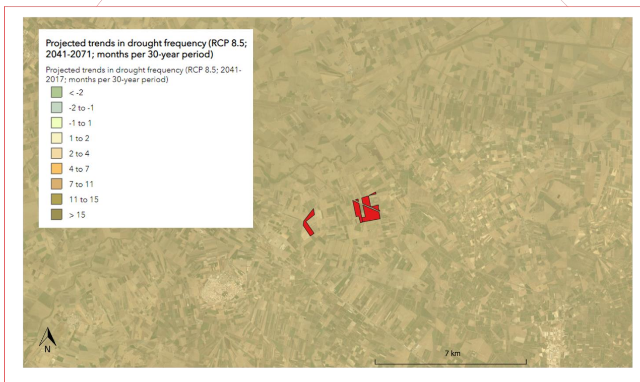
Figura 6. Previsione della frequenza di eventi siccitosi in 30 anni per lo scenario RCP 8.5 ( Climate-ADAPT ). L'area di studio è indicata in rosso.
