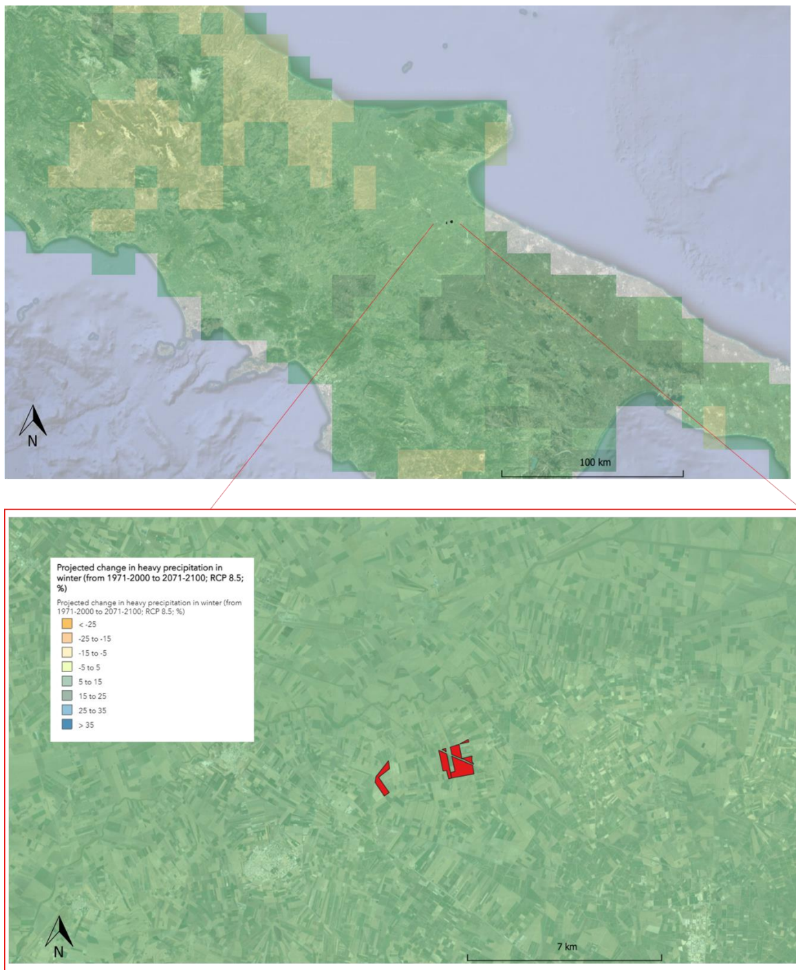
Figura 5. Previsione dei cambiamenti nelle precipitazioni intense (in %) in inverno dal 1971-2000 al 2071-2100 per lo scenario RCP 8.5 ( EURO-CORDEX ). L'area di studio è indicata in rosso.
