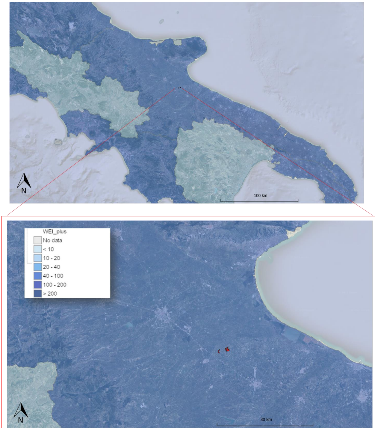
Figura 7. Indice di sfruttamento della risorsa idrica (WEI+). Fonte: European Environment Agency (EEA) 20
