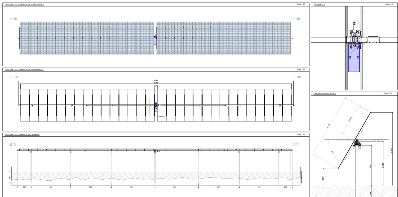
Figura 1 – Particolari costruttivi tracker
