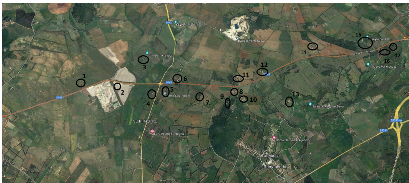
Figura 8 – Presenza recettori prossimi al cavidotto MT
