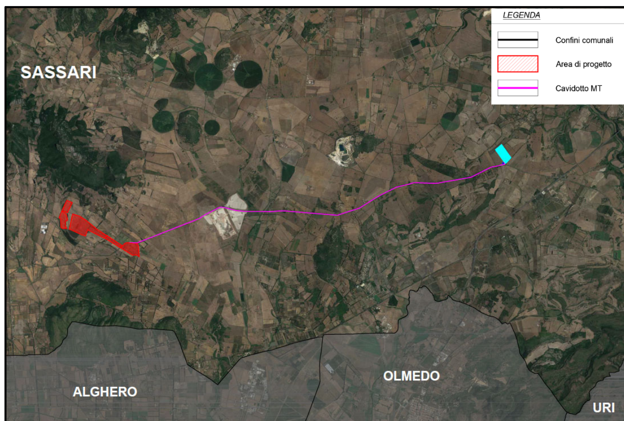
Figura 1 - Estratto ortofoto area parco agrivoltaico
