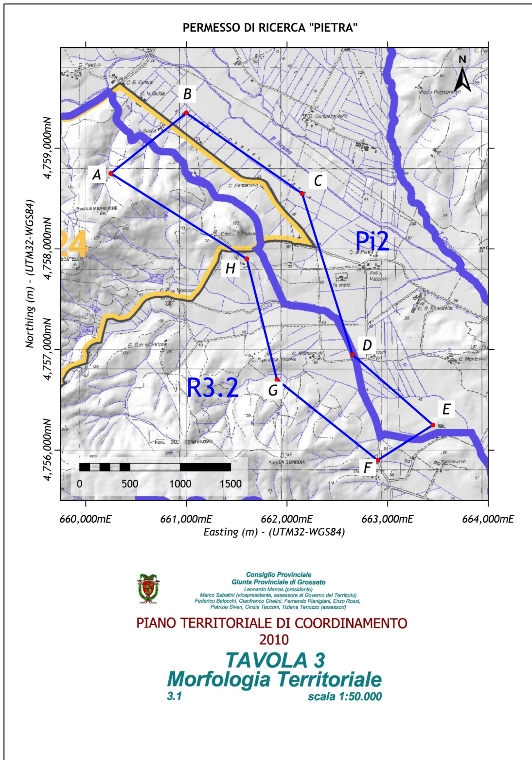
TAVOLA 4.2.a – Carta Morfologia Territoriale (da Tavola 3 del PTC GR)
