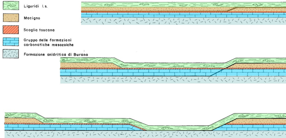
Figura 2.3.a - Schema semplificato del meccanismo di formazione della "Serie Toscana ridotta" (da Bertini et al., 1991).
