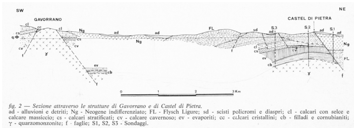
Figura 2.3.d - Sezione attraverso le strutture di Gavorrano e di Castel di Pietra (da Arisi Rota & Vighi, 1974).
