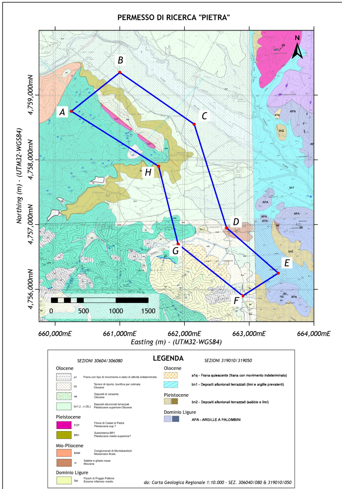
TAVOLA 2.3.a – Carta Geologica (da Progetto CARG 1:10,000, Regione Toscana)
