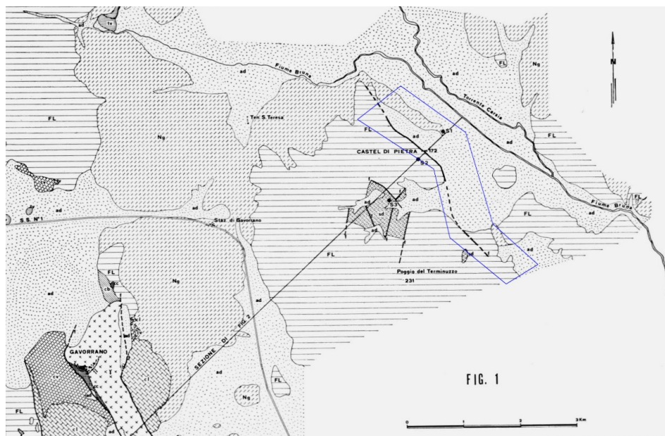
Figura 2.3.c - Carta Geologica della zona tra Gavorrano e Castel di Pietra (da Arisi Rota & Vighi, 1974).
