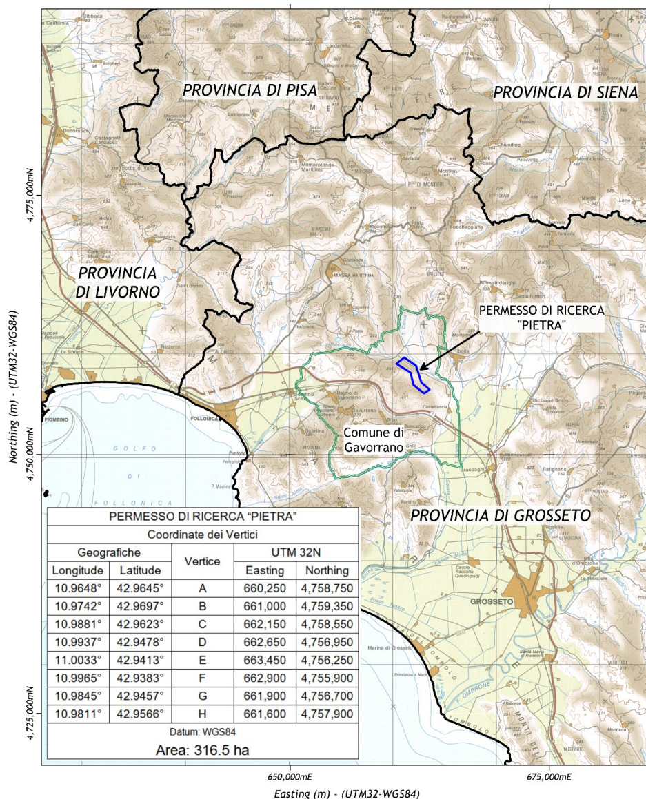
Figura 2.1.a – Inquadramento cartografico dell'area del Permesso di Ricerca "Pietra"
